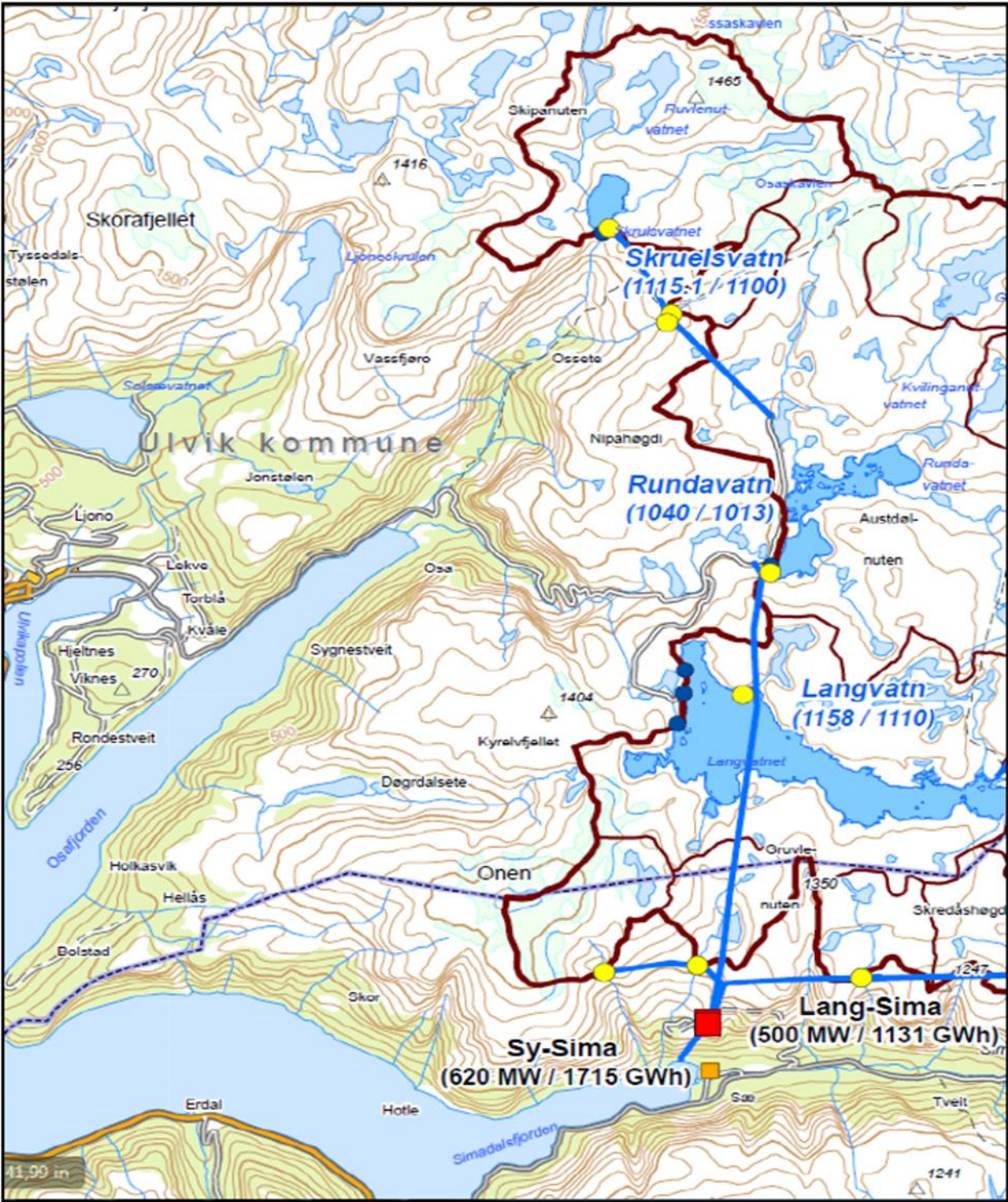
Vedlegg 1c. Eidfjord Nord-utbyggingen – oversikt over Lang-Sima-overføringen
