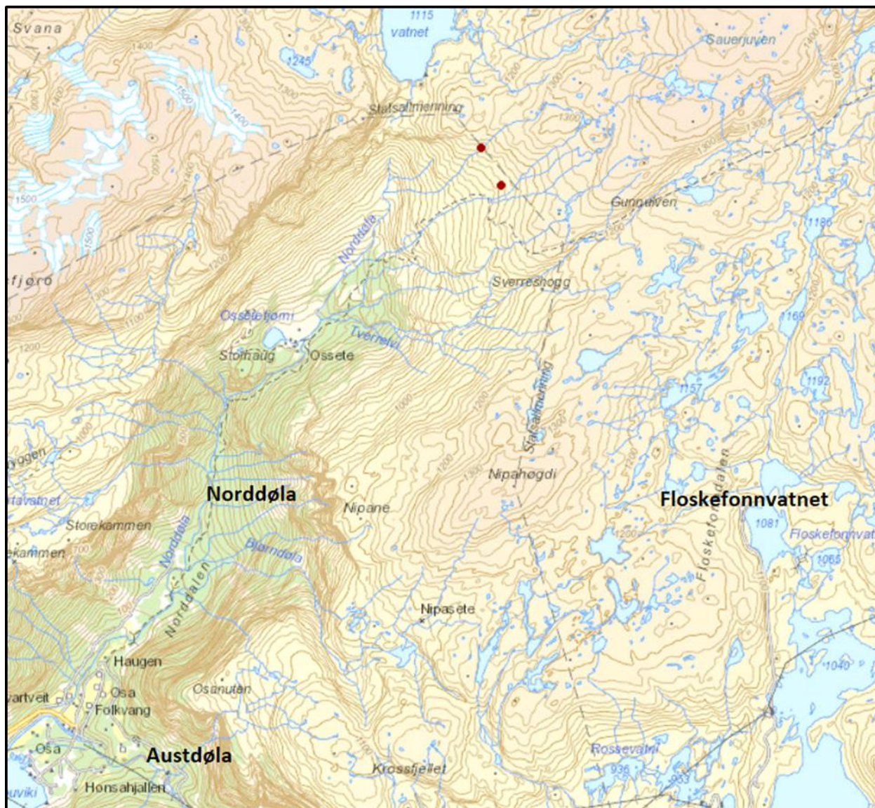
Vedlegg 1a. Oversiktskart over tiltaksområdet. Inntak i Våtekleivbekkane markert rød prikker.
