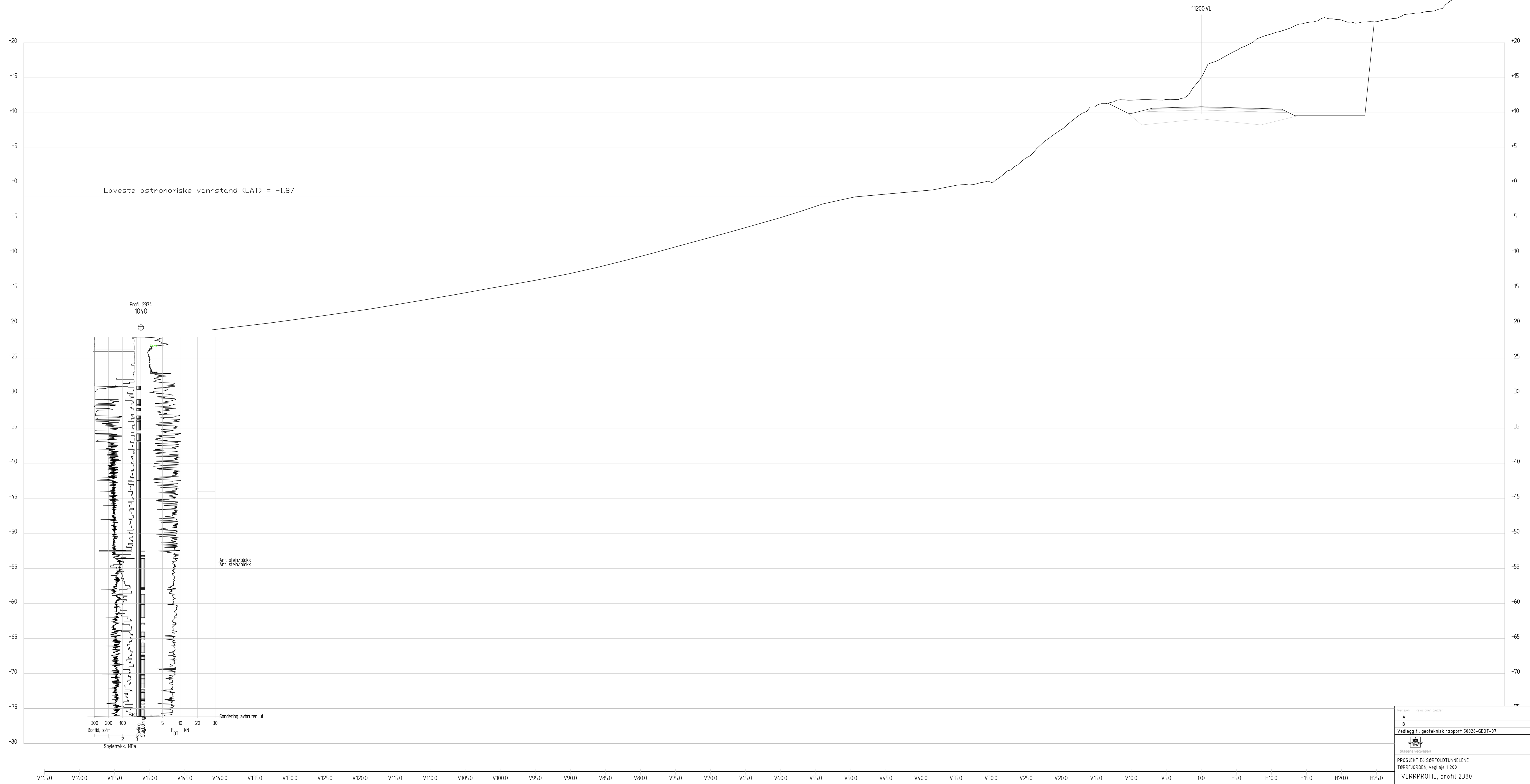
Profil 2380 1 : 200
