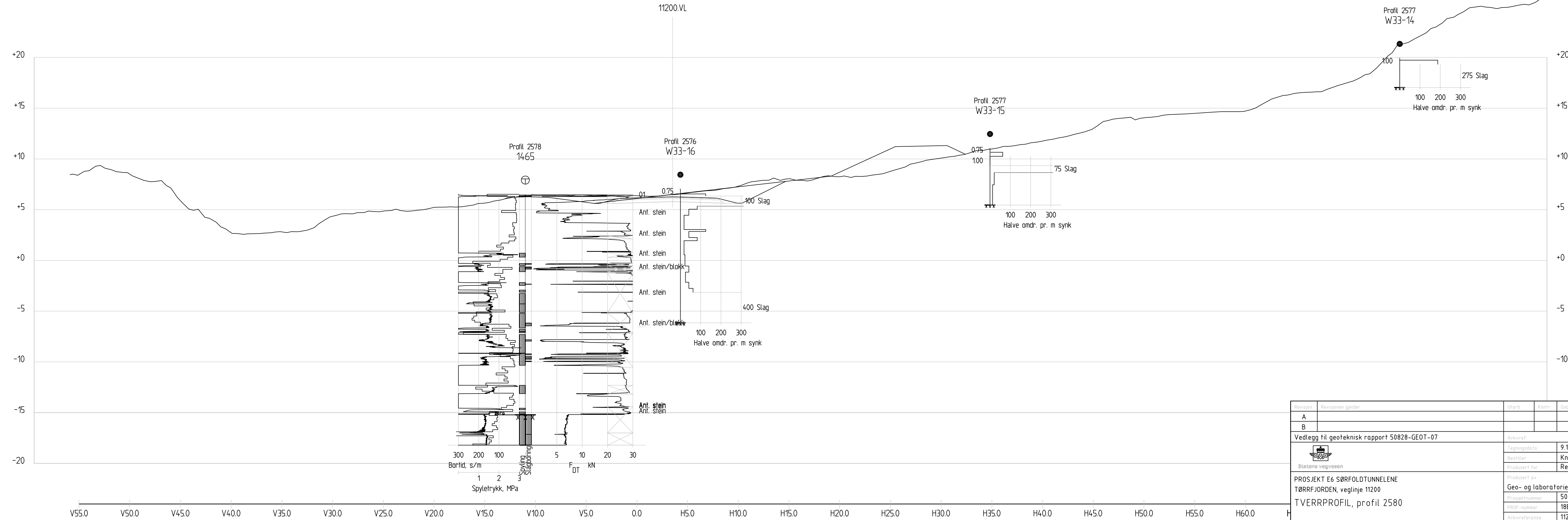
Profil 2580 1 : 200
