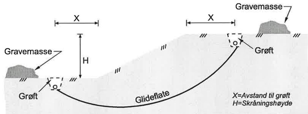
Figur C1 Ved graving av grøfter i fot og topp av bratte leirskråninger bør gravmassene plasseres vekk fra skråningen.
