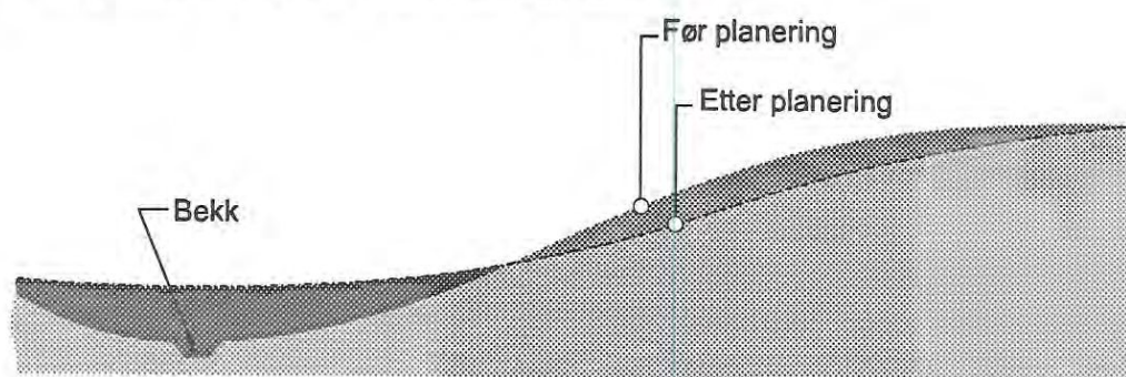
Figur C4 Planering ved oppfylling av dalbunnen forbedrer stabiliteten
