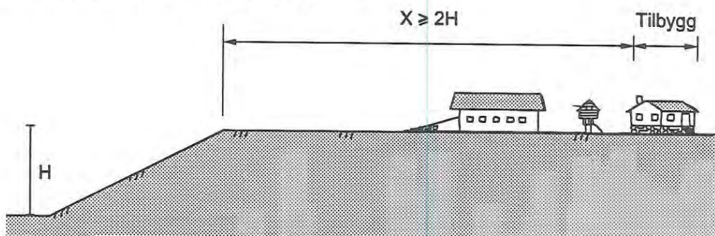
Figur C10 Ny bebyggelse i ravinert leirterreng
