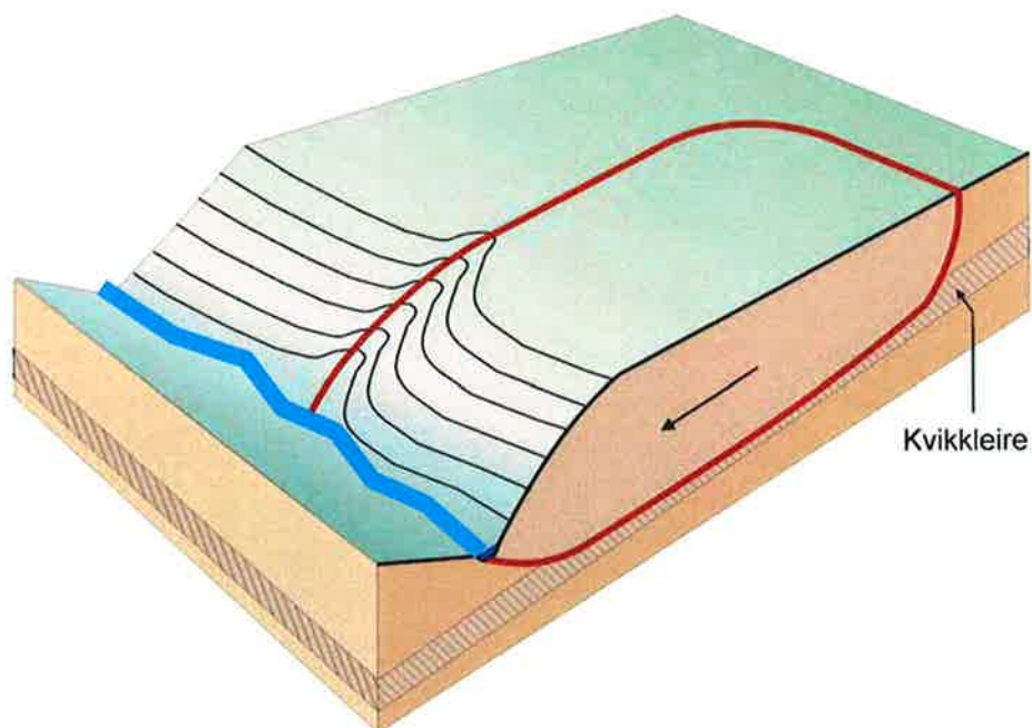
Figur 2.3 Flakskred, utløst ved progressiv bruddutvikling i sprøbruddmateriale
