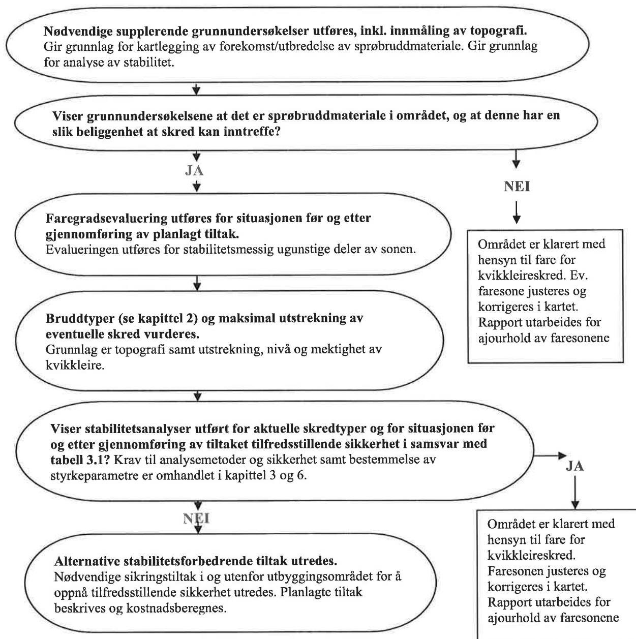
Figur 4.2 Flytskjema for vurdering av reell skredfare
