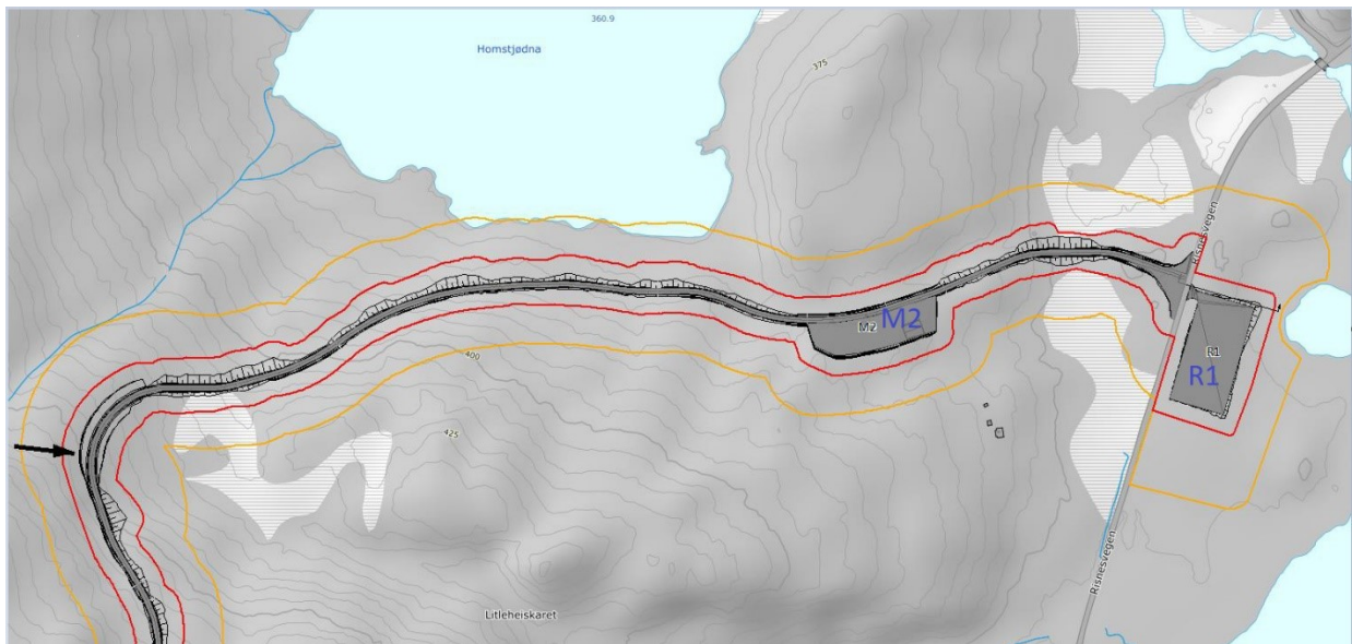
Figur 1: Fra søknad av 17.03.2020. Buheii Vinkraft AS søker delgodkjenning opp til pilen på adkomstveien, samt riggområde øst for Fv465. Rød linje markerer ytre inngrepsgrense, og gul linje arealbruksgrense.
