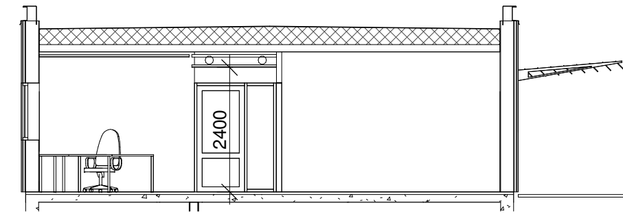
Snitt 1 : 100
