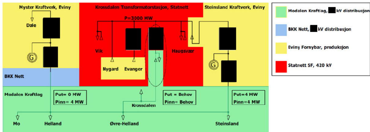
Figur 6 Forenkla oversiktsskjema med distribusjonsnett i Modalen med eksterne grensesnitt og foreslått ny tilkøpling ved nye Krossdalen transformatorstasjon
