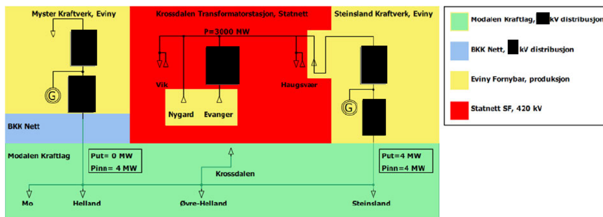
Figur 5 Forenkla oversiktsskjema med distribusjonsnett i Modalen med eksterne grensesnitt og eigarskap etter omsøkt tiltak
