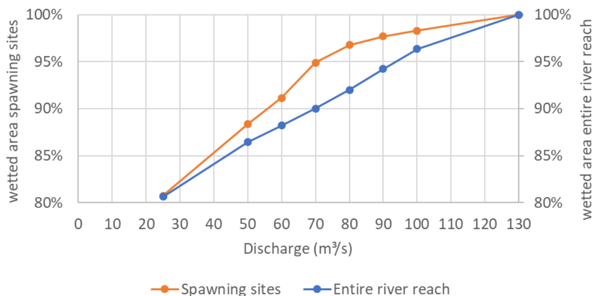
Figur 9. Prosentvis vanndekt areal i forhold til vannføring i Otra for gyteområder (oransje linje) og hele elvearealet (blå linje). For hele elvearealet er det en tilnærmet lineær sammenheng mellom vannføring og vanndekt areal. For gyteområdene er det et tydelig knekkpunkt ved 70 m³/s. Det er en økt tørrlegging av gyteområdene med vannføringer lavere enn 70 m³/s enn sammenlignet med vannføringer over 70 m³/s. Figuren er hentet fra Flödl & Hauer 2023, vedlagt appendiks.
