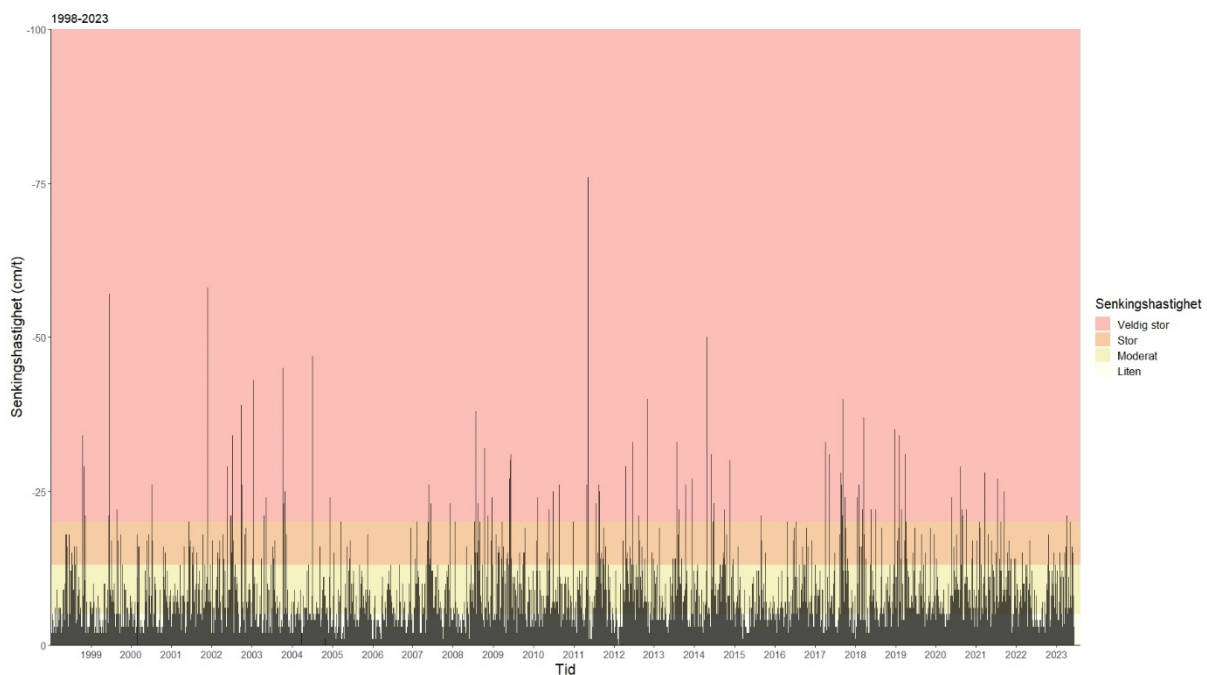
Figur 6. Senkningshastigheter, dvs. reduksjon i vannstand fra en time til neste i perioden 1998 - 2023 nedstrøms Vigeland kraftverk. Fargeskalaen indikerer grenseverdier for klassifisering av effekt fra Bakken mfl. (2016).
