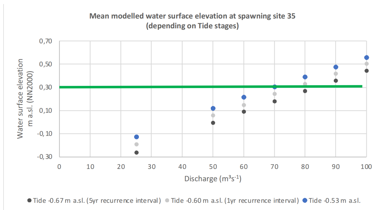
Figur 12. Modellert vannstandsnivåer ved Stavsøyra ved ulike vannføringer og havnivåer på hhv. -0.67 m (svarte punkter), -0.60 m (grå punkter) og -0.53 m under NN2000. Grønn linje angir vannstandsnivå på Stavsøyra som dekker gyteområdet helt med vann. Figuren er hentet fra Flödl & Hauer 2023, vedlagt appendiks.
