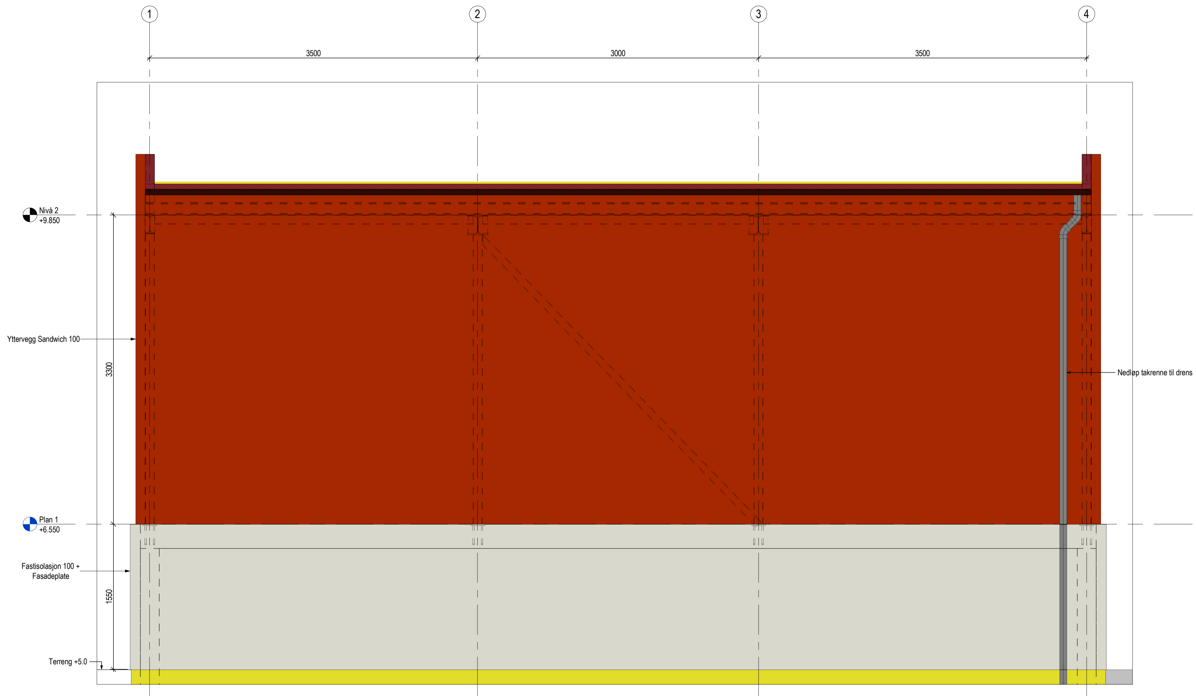
Fasade Vest 1:25
