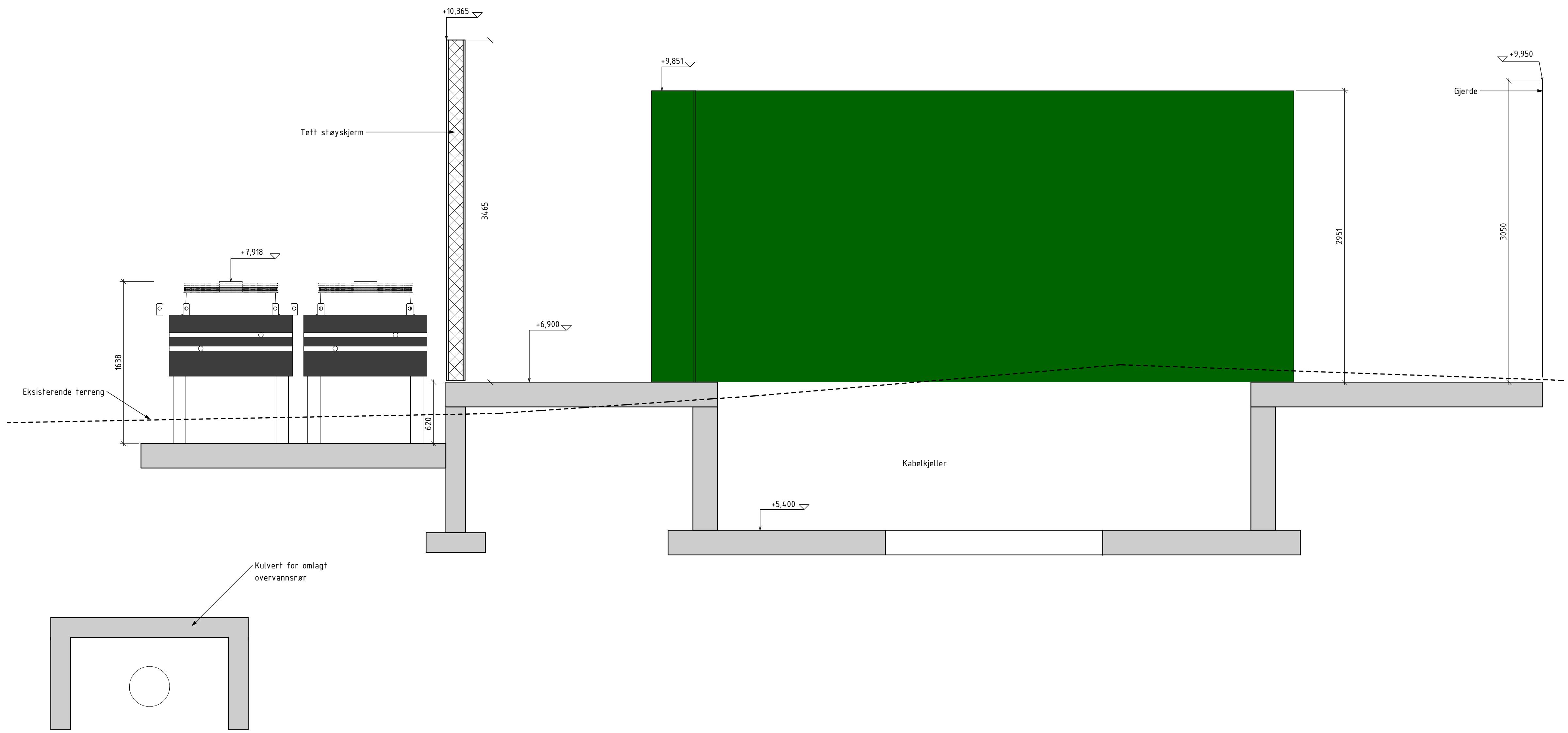
Snitt F4 1: 25
