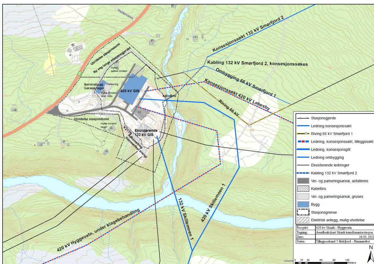
Figur 7. Arealbrukskart Skaidi transformatorstasjon med ledningsinnføringer.
