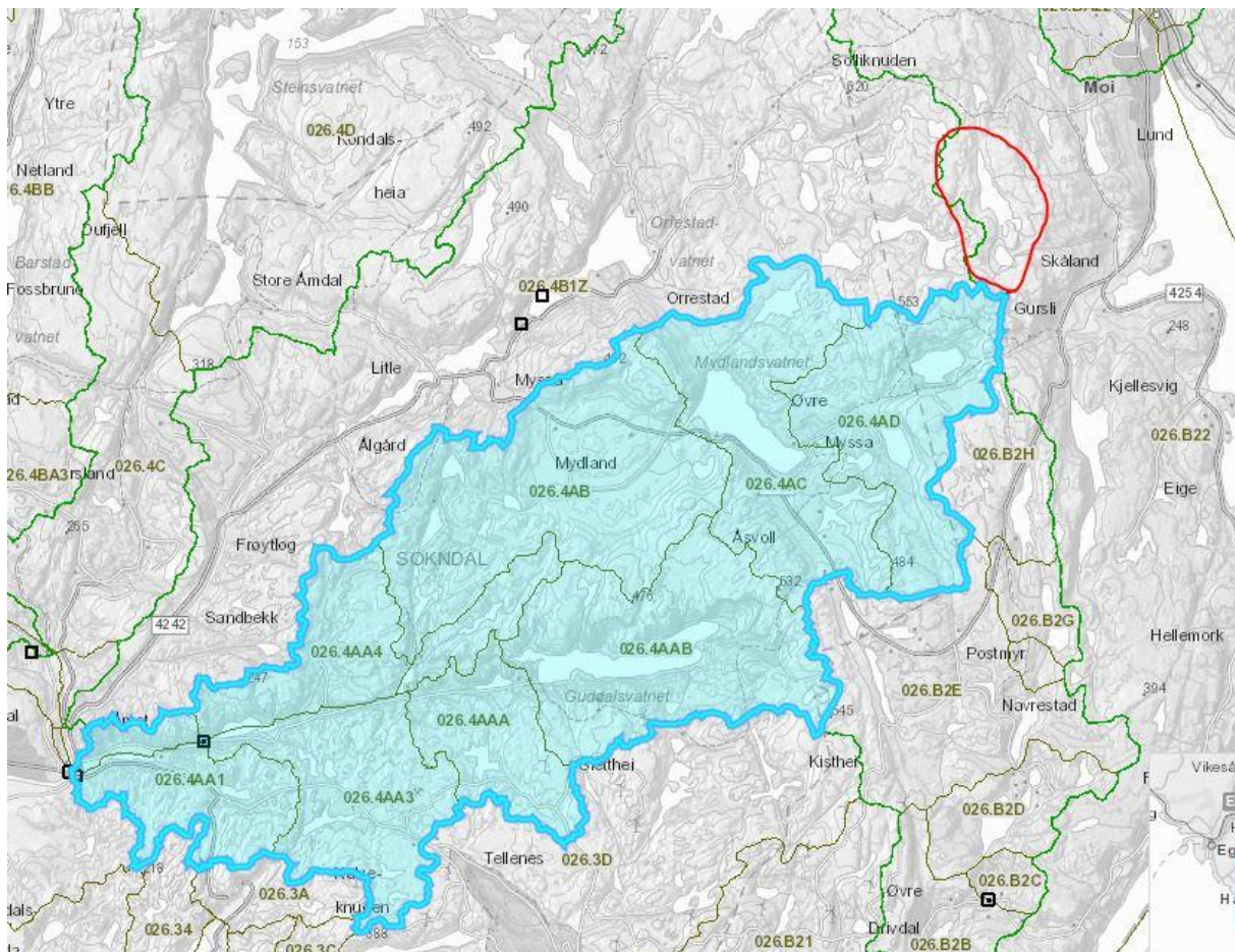
Figur 2b. Nedbørsfelt for Refsvatn. Nedbørsfelt Storeli kraftverk indikert med rød strek (se fig. 2a)
