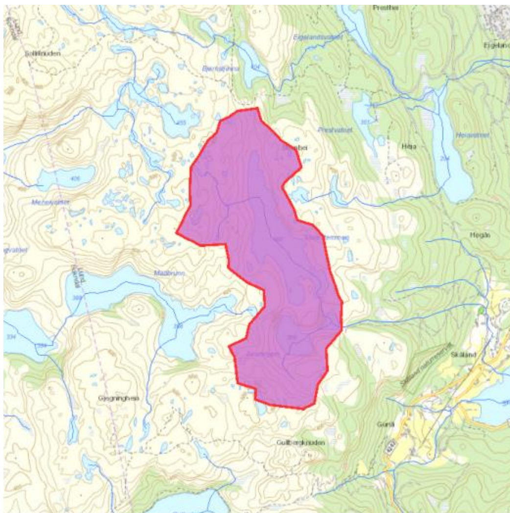
Figur 2a. Nedbørsfelt for Storeli kraftverk
