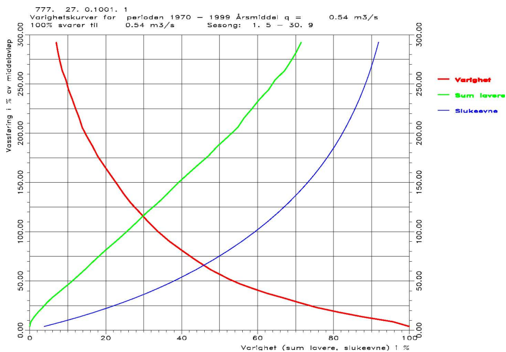
Figur 9. Varighetskurve for sommersesongen (1/5 – 30/9).
