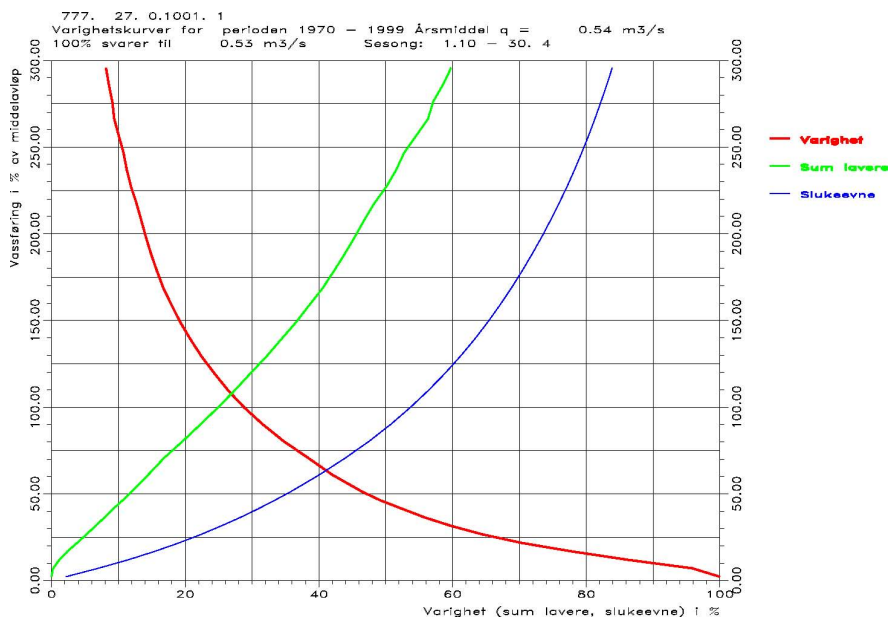
Figur 10. Varighetskurve for vintersesongen (1/10 – 30/4).
