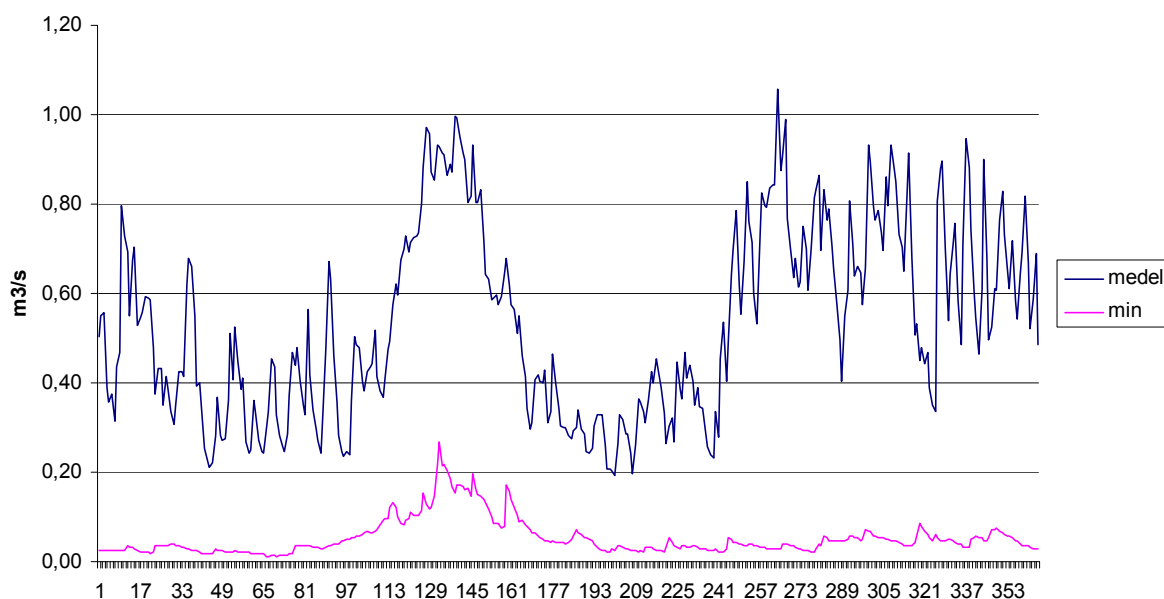
Figur 3. Plott som viser middel/median- og minimumsvannføringer (døgndata). 13
