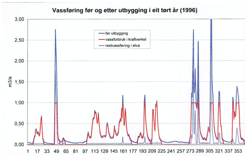
Figur 6. Plott som viser vannføringsvariasjoner i et tørt (åååå) år (før og etter utbygging). 16
