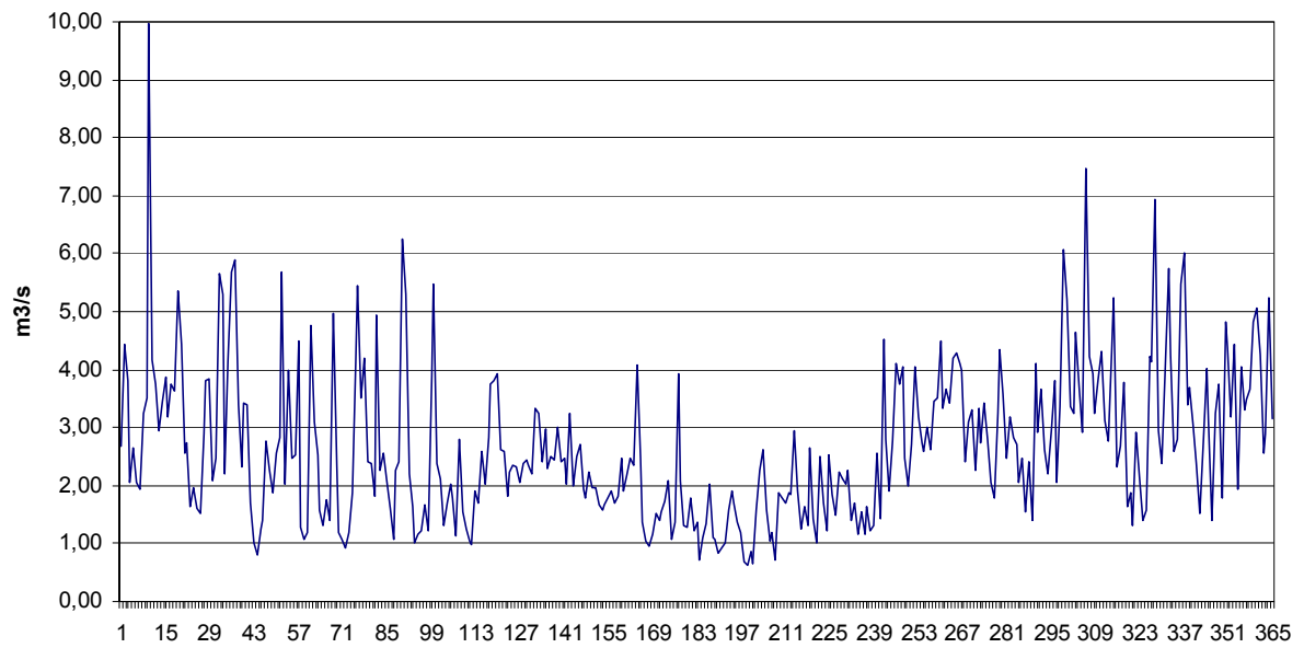
Figur 4. Plott som viser maksimumsvannføringer (døgndata). 14
