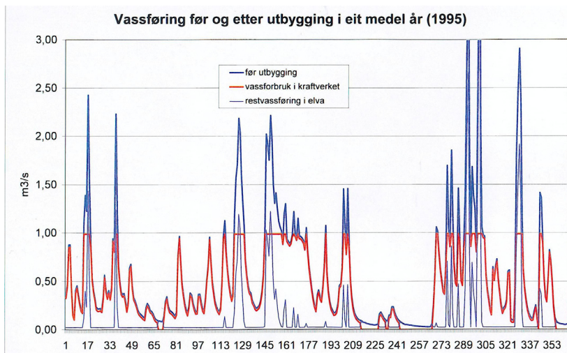
Figur 7. Plott som viser vannføringsvariasjoner i et middels (åååå) år (før og etter utbygging). 17
