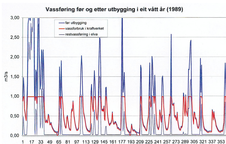
Figur 8. Plott som viser vannføringsvariasjoner i et vått (åååå) år (før og etter utbygging). 18
