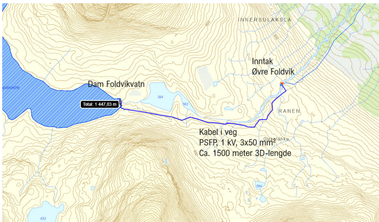
Figur 1: Oversiktskart med omsøkt trasé for 1 kV jordkabel mellom hovedinntaket til Øvre Foldvik kraftverk og dam Foldvikvatn. Kabelen er planlagt lagt i veikropp til en eksisterende vei som Småkraft planlegger å oppgradere i forbindelse med utbyggingen.
