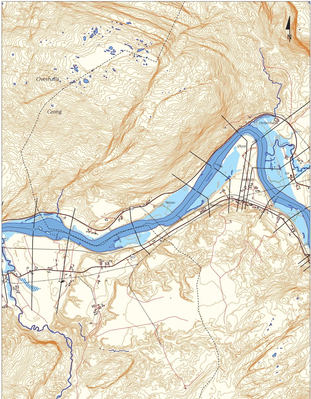
Figur 4.3 Flomsonekart for 10-årsflom, Valskrå
