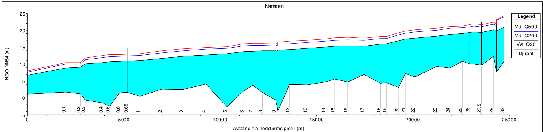
Figur 3.2 Beregnede vannstander for 20-, 200- og 500-årsflom i Namsen ved Grong, i Namsen og Sanddøla
