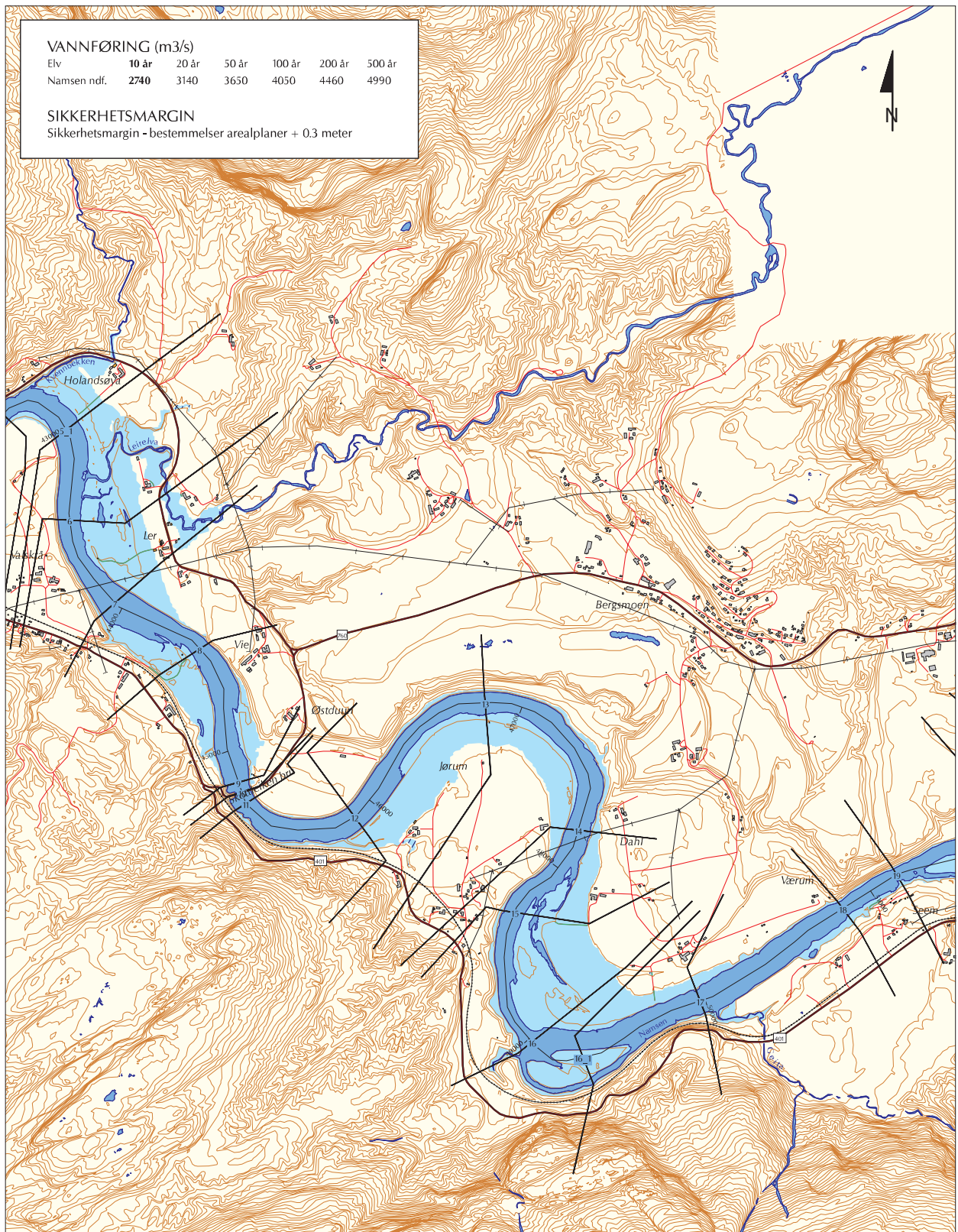
Figur 4.4 Flomsonekart for 10-årsflom, Bergsmo
