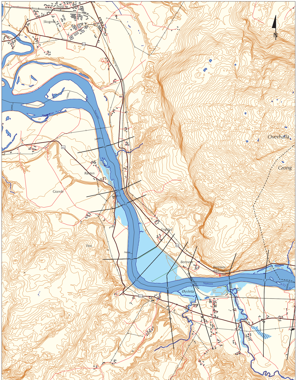
Figur 4.2 Flomsonekart for 10-årsflom, Øysletta
