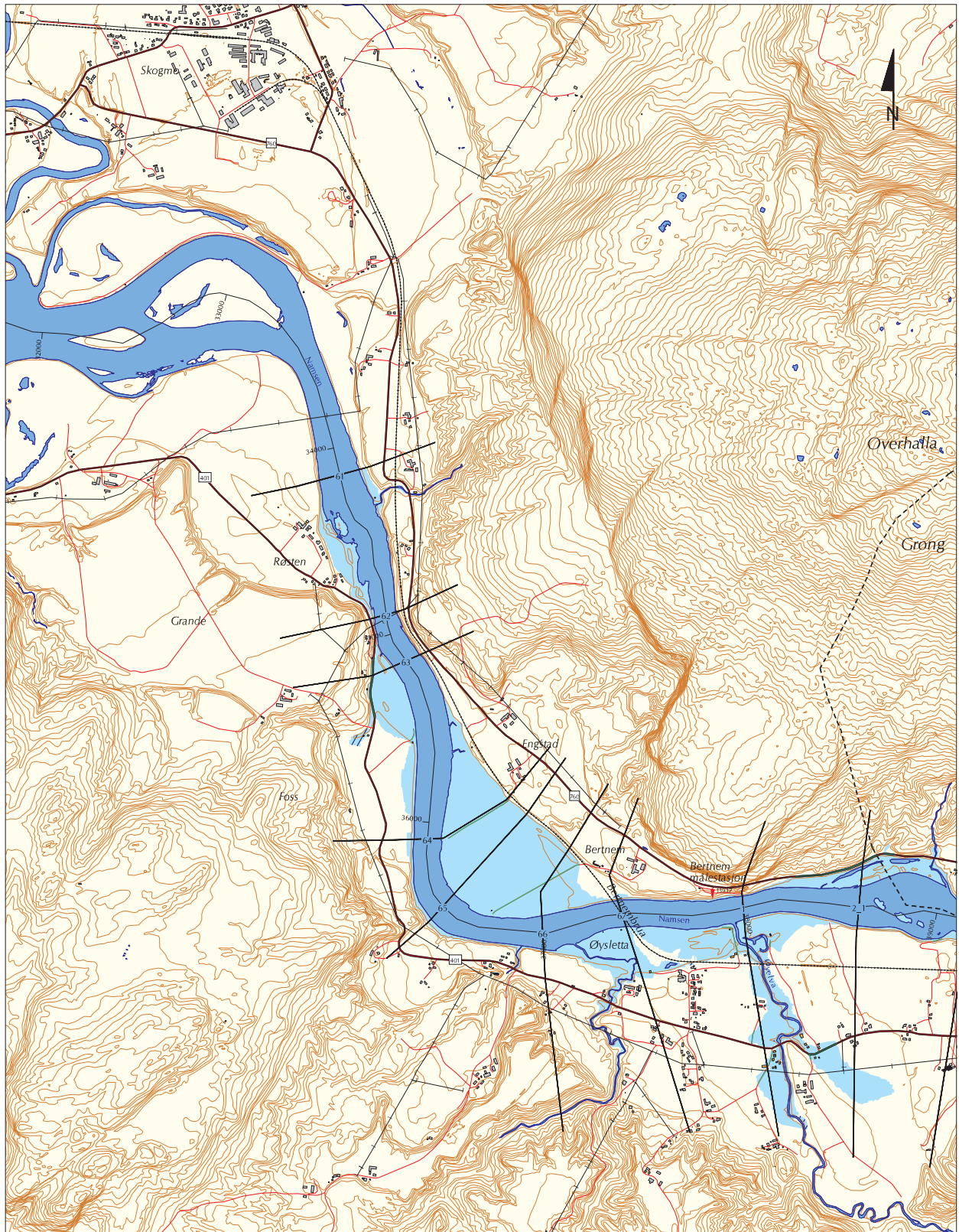
Figur 4.6 Flomsonekart for 50-årsflom, Øysletta
