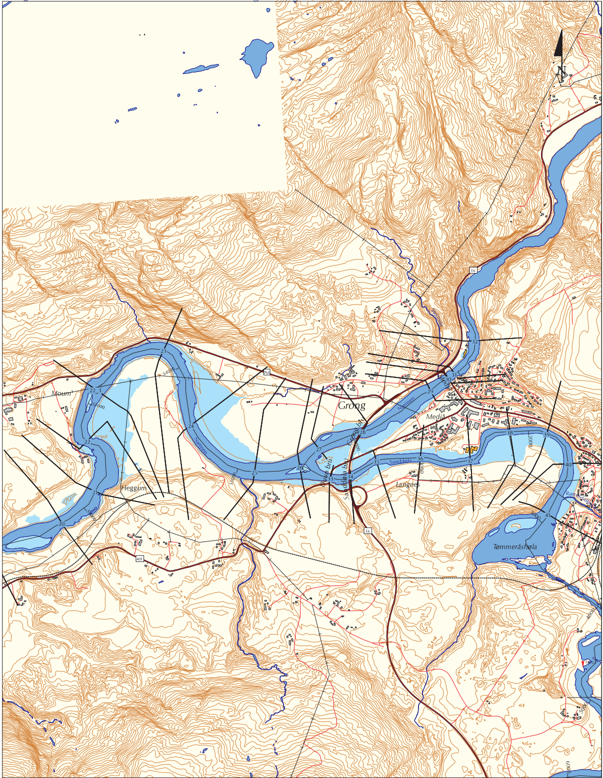
Figur 4.5 Flomsonekart for 10-årsflom, Grong sentrum
