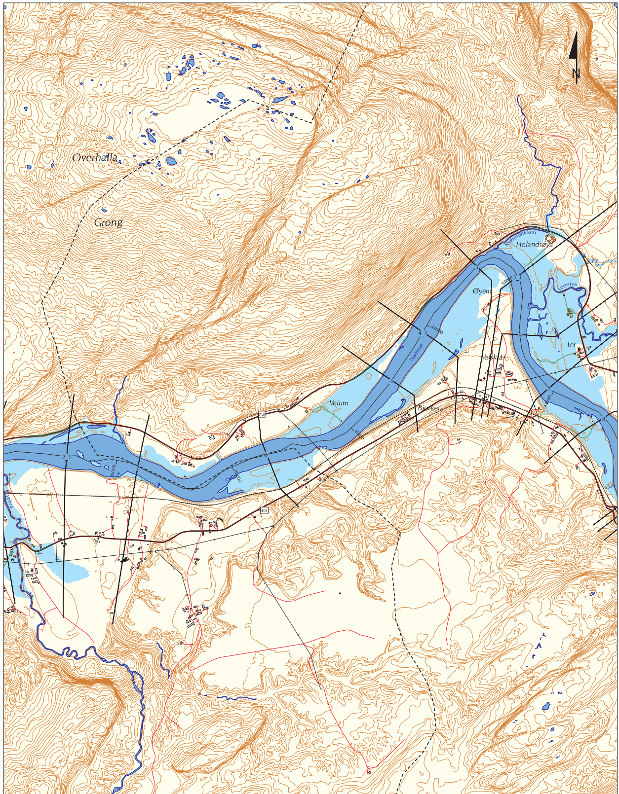
Figur 4.7 Flomsonekart for 50-årsflom, Valskrå
