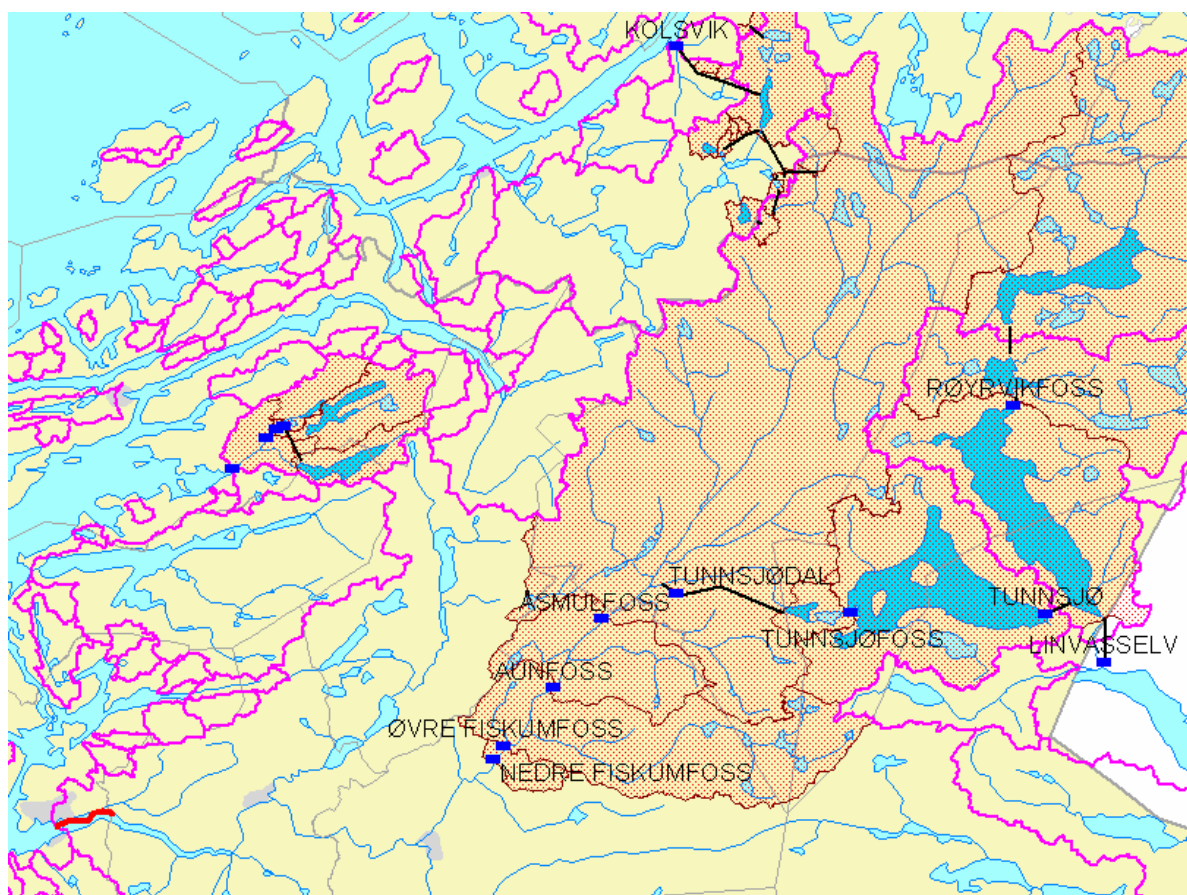
Figur 2.1 Kart over Namsens nedbørfelt med inntegnet kraftstasjoner og overføringer
