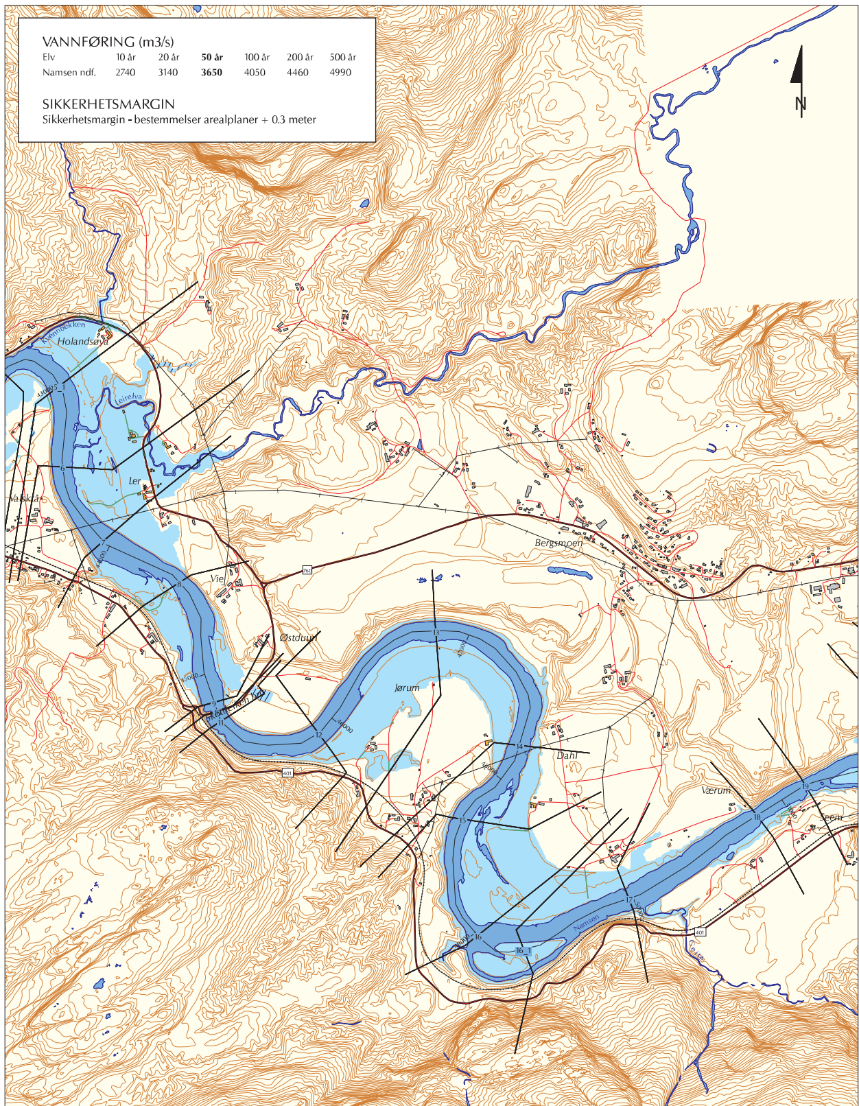
Figur 4.8 Flomsonekart for 50-årsflom, Bergsmo
