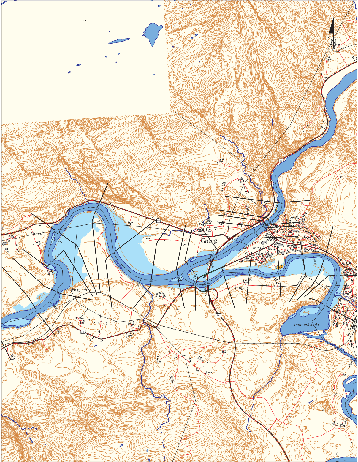
Figur 4.9 Flomsonekart for 50-årsflom, Grong sentrum
