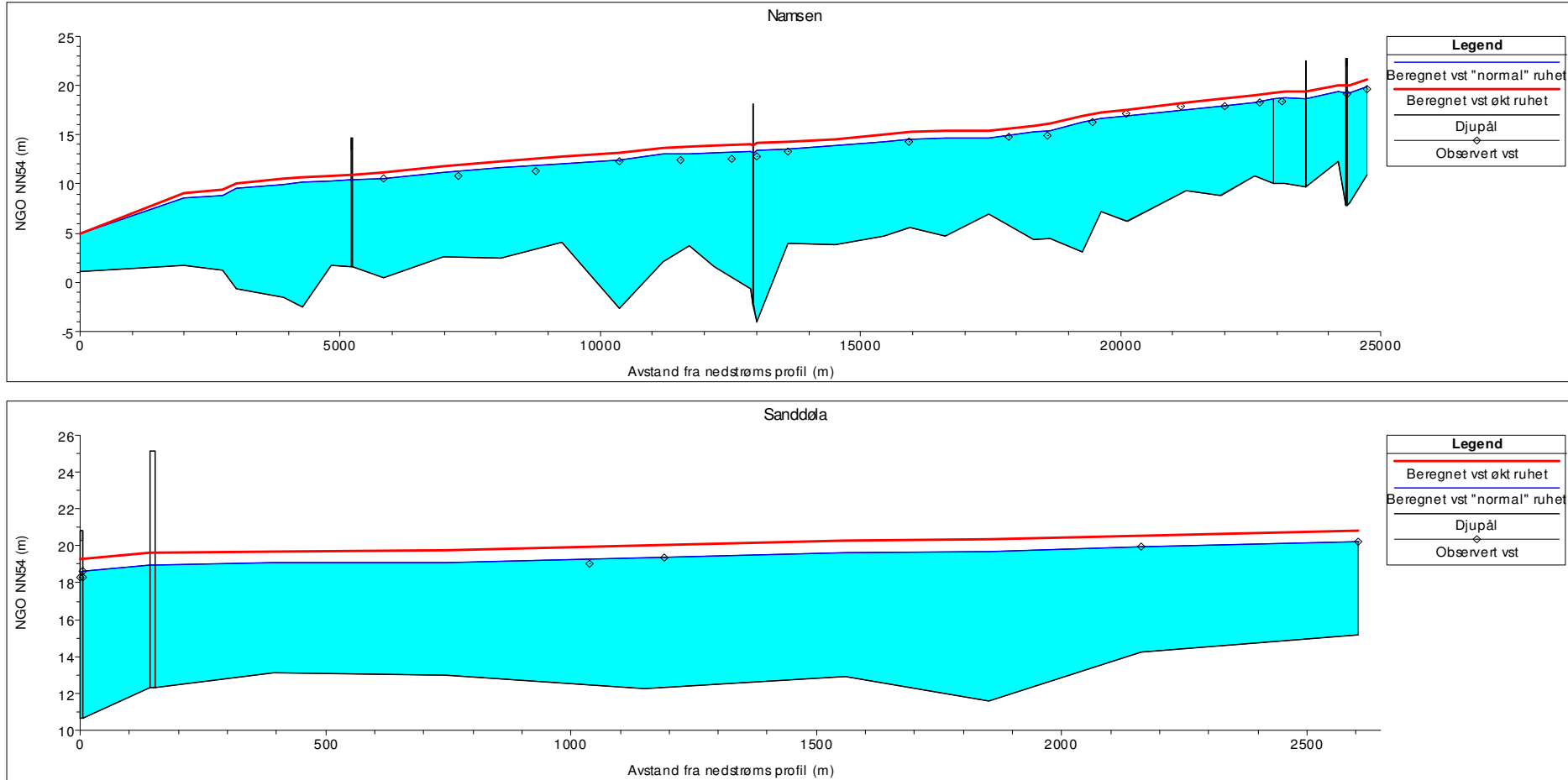
Figur 3.1 Virkning av å øke ruheten med 20 % for en 200-årsflom i Namsen ved Grong, både i Namsen og Sanddøla
