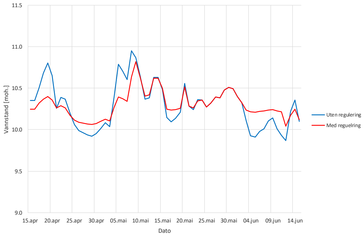
Vannstandskurver Litlevatnet i eggerperioden 15/4 - 15/6 - Vått år
