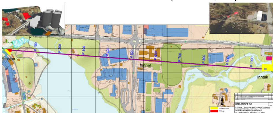
Skissert plan og profil tilløpstunnel, hentet fra konsesjonssøknad.
