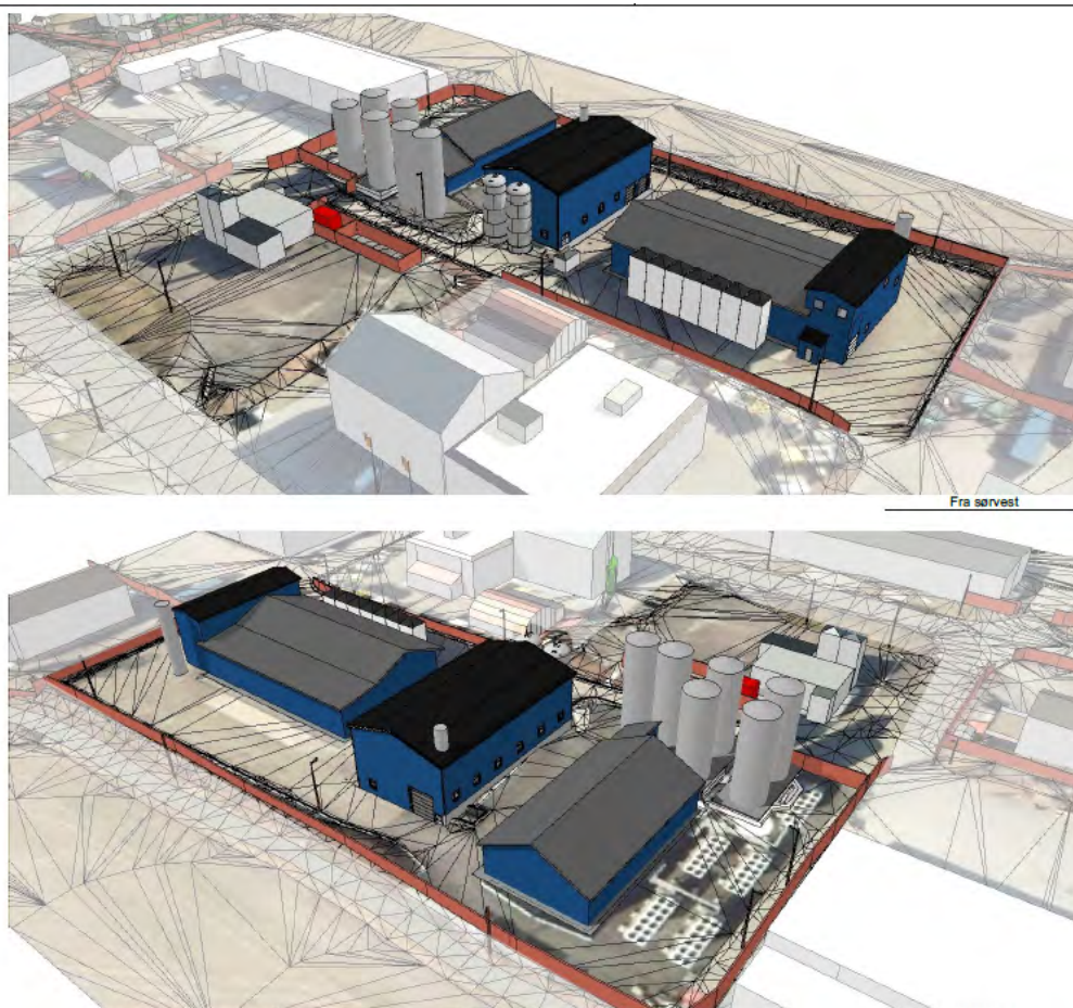
Figur 2 – Tegning av ny pelletsbasert varmesentral på Drømtorp
