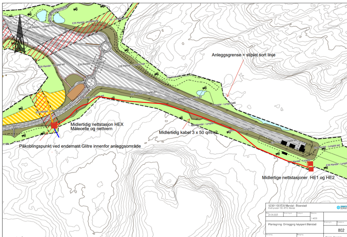
Figur 3: Plassering av netstasjoner og høyspentkabel i Vråheiatunnelen, markert i rødt. Kilde: Hæhre Entreprenør sin konsesjonssøknad av 22. oktober 2025.
