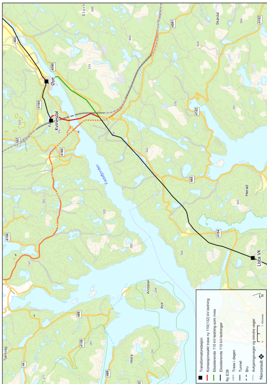
Figur: Kartet viser konsesjonsgitt trasé for 132 kV Lista vindpark—Kvinesdal koblingsstasjon. Den nye forbindelsen vises i rødt. Eksisterende forbindelse til Øye som skal rives vises i grønt. Kilde: Glitre Nett.
