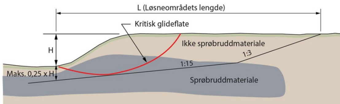
Figur 3-15: Definisjon av løsnakeområde for retrogressive skred iht. NGI-metoden[5].
