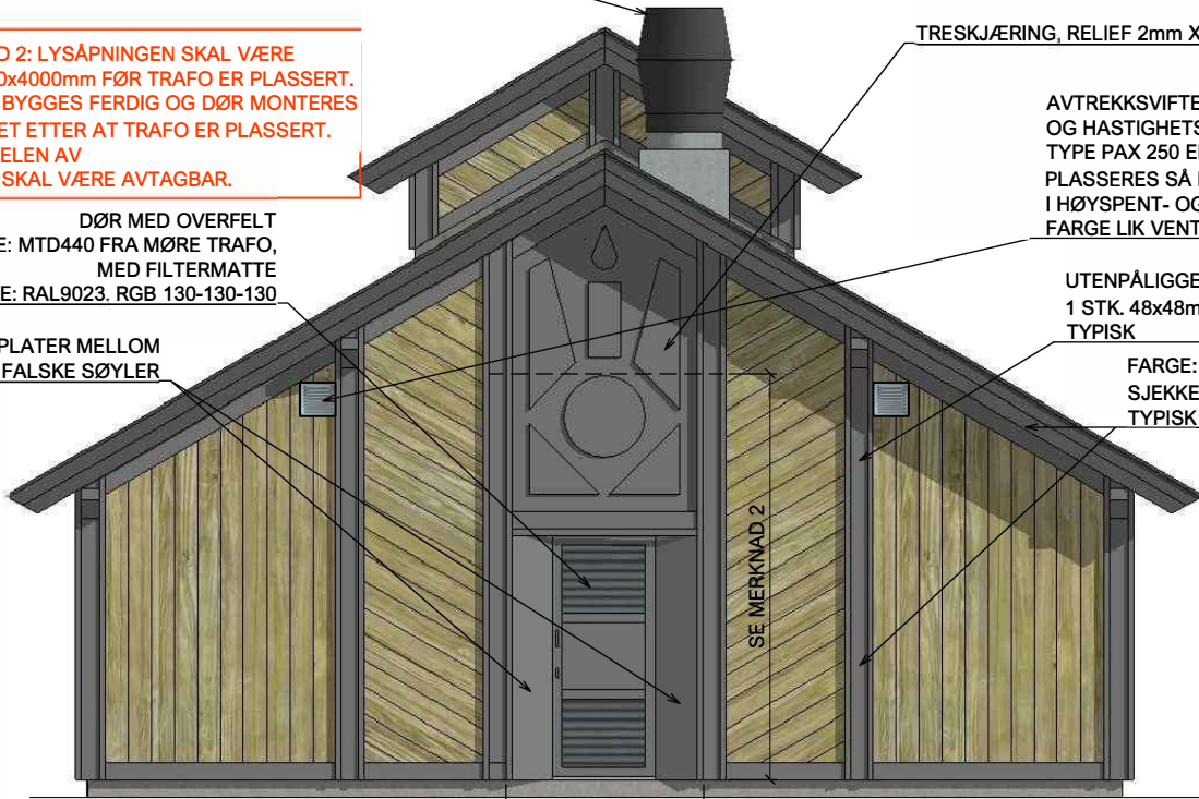
FASADE SØRØST
