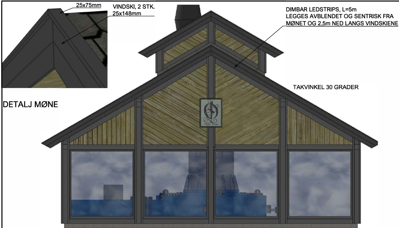
FASADE SØRØST
