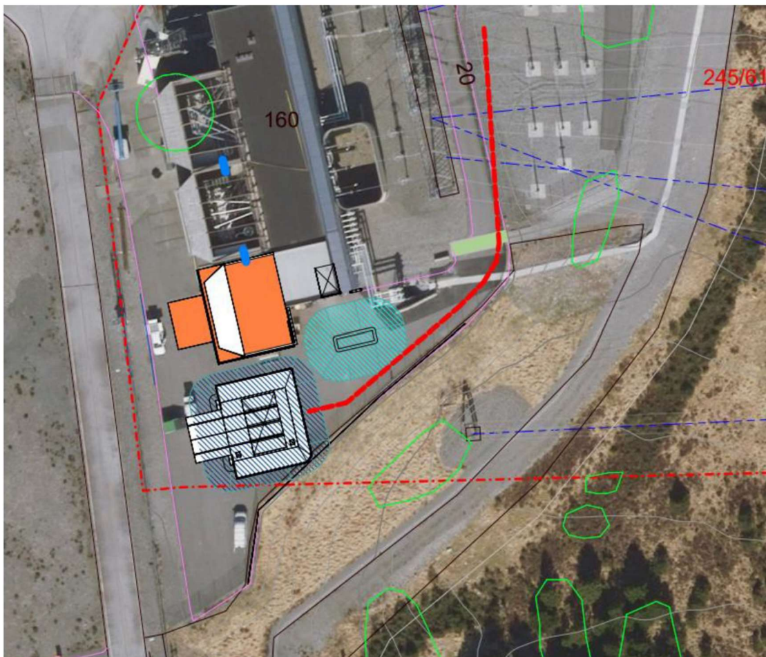
Ny transformator i Kollsnes stasjon (oransje felt)
