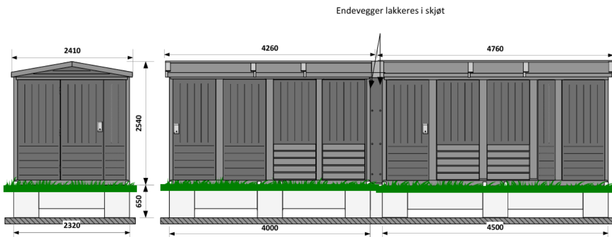
Figur 2. Fasade og spesifikasjoner på nettstasjon. Kilde: Teslas søknad av 16. februar 2026.
