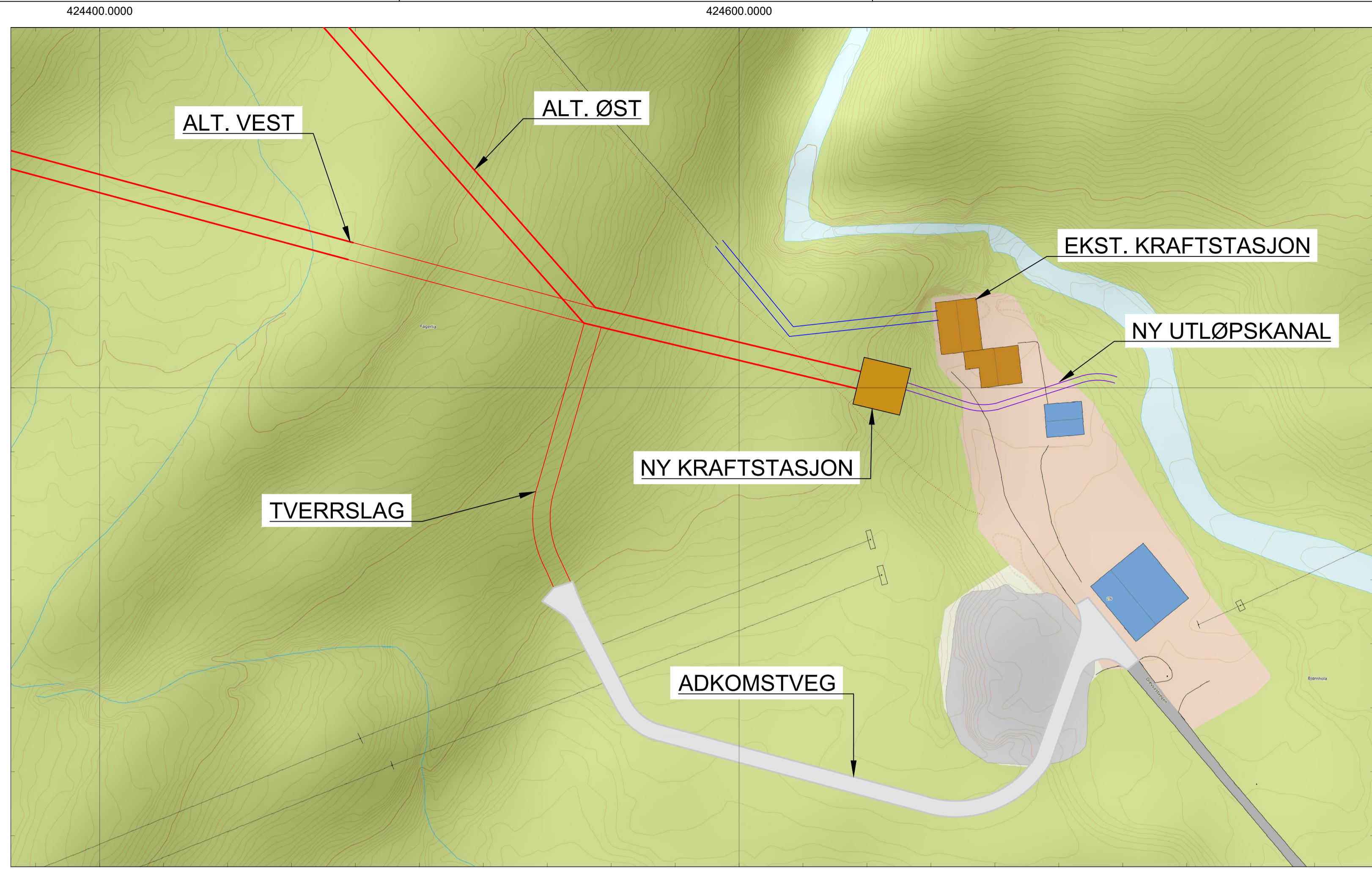
KALDÅGA KRAFTVERK - KRAFTSTASJONSOMRÅDE - STASJON I DAGEN - PLAN 1:1000
