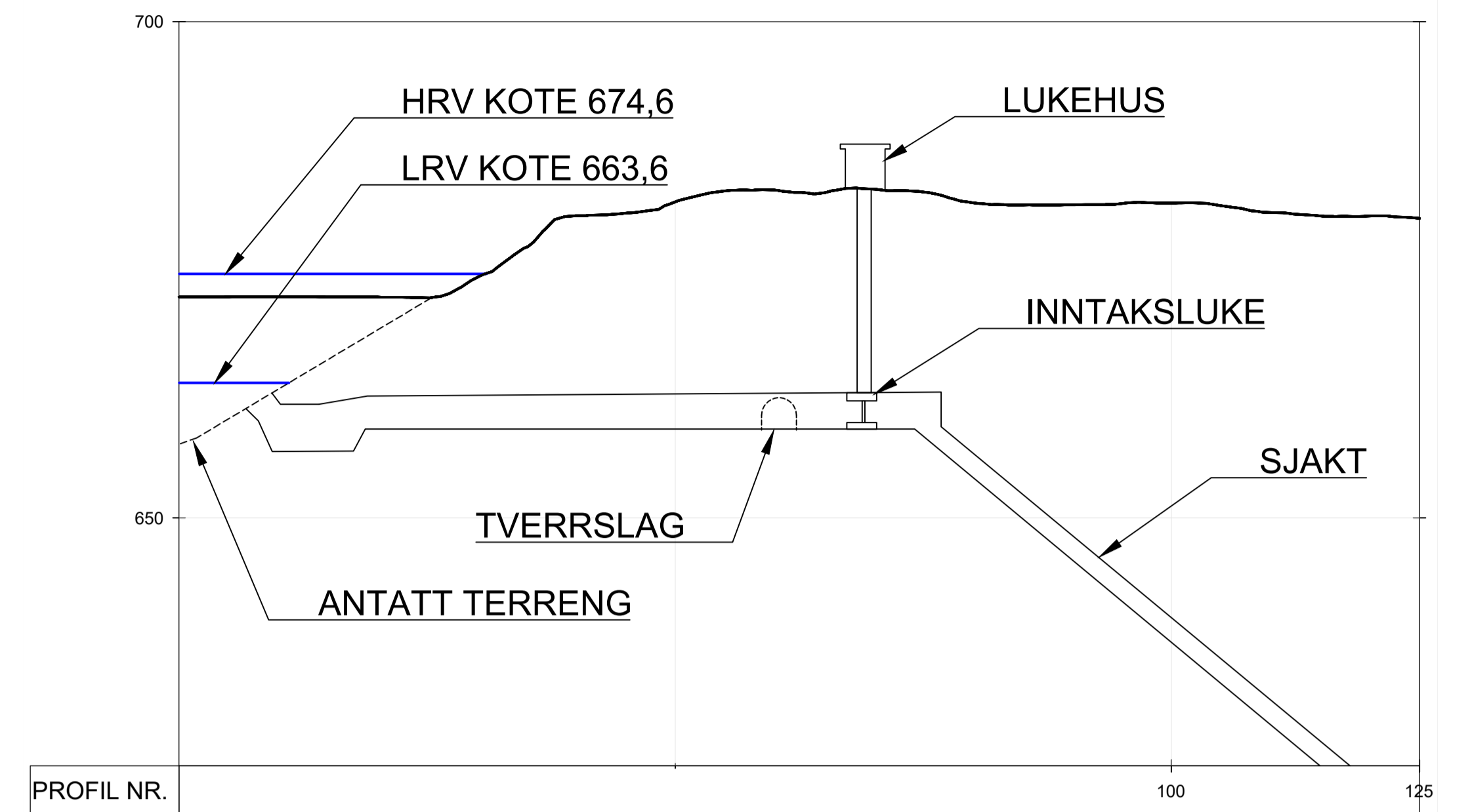
KALDÅGA KRAFTVERK - NYTT INNTAK ENVATN - LENGDESNITT 1:500
