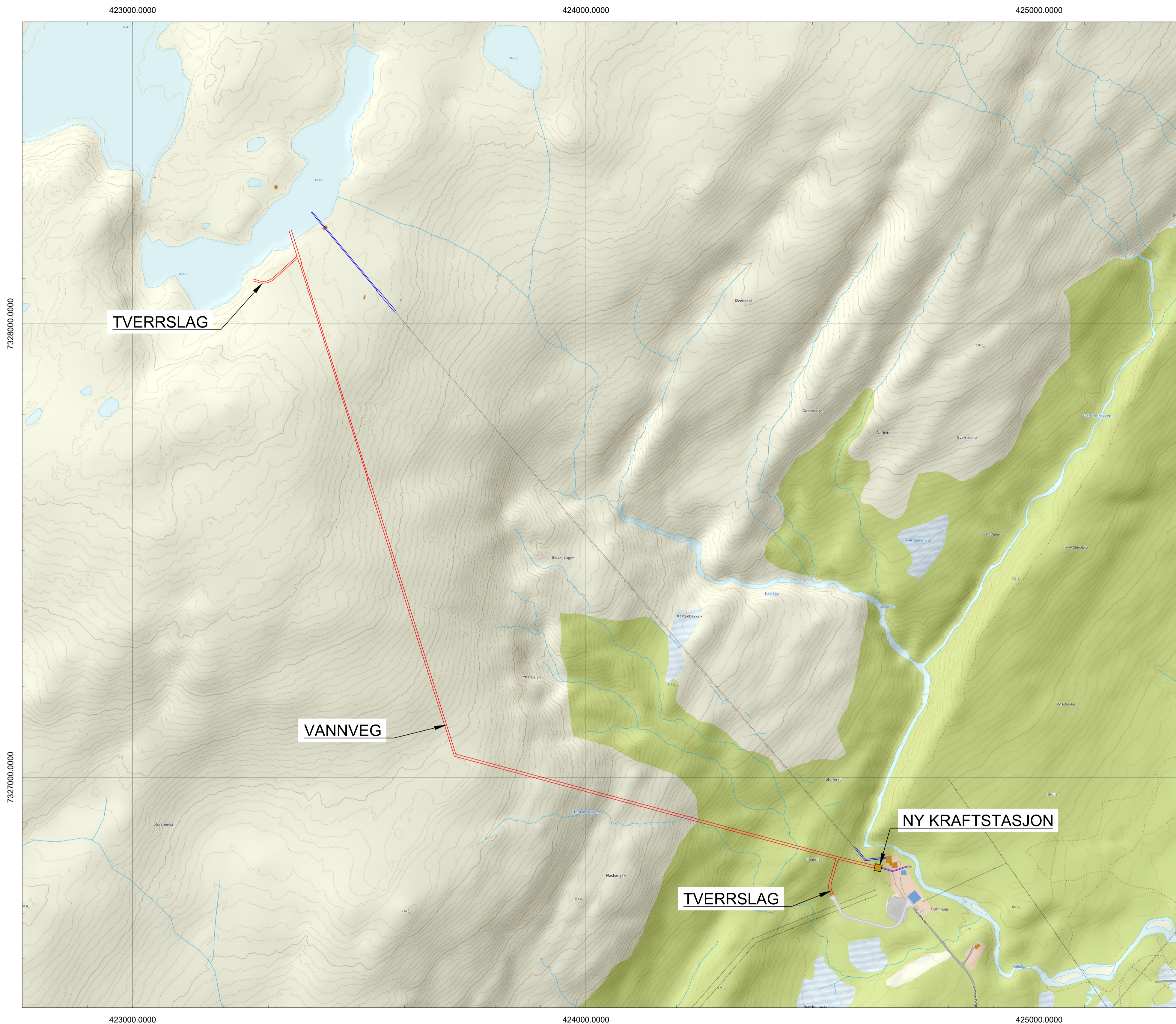
KALDÅGA KRAFTVERK - STASJON I DAGEN - PLAN 1:5 000
