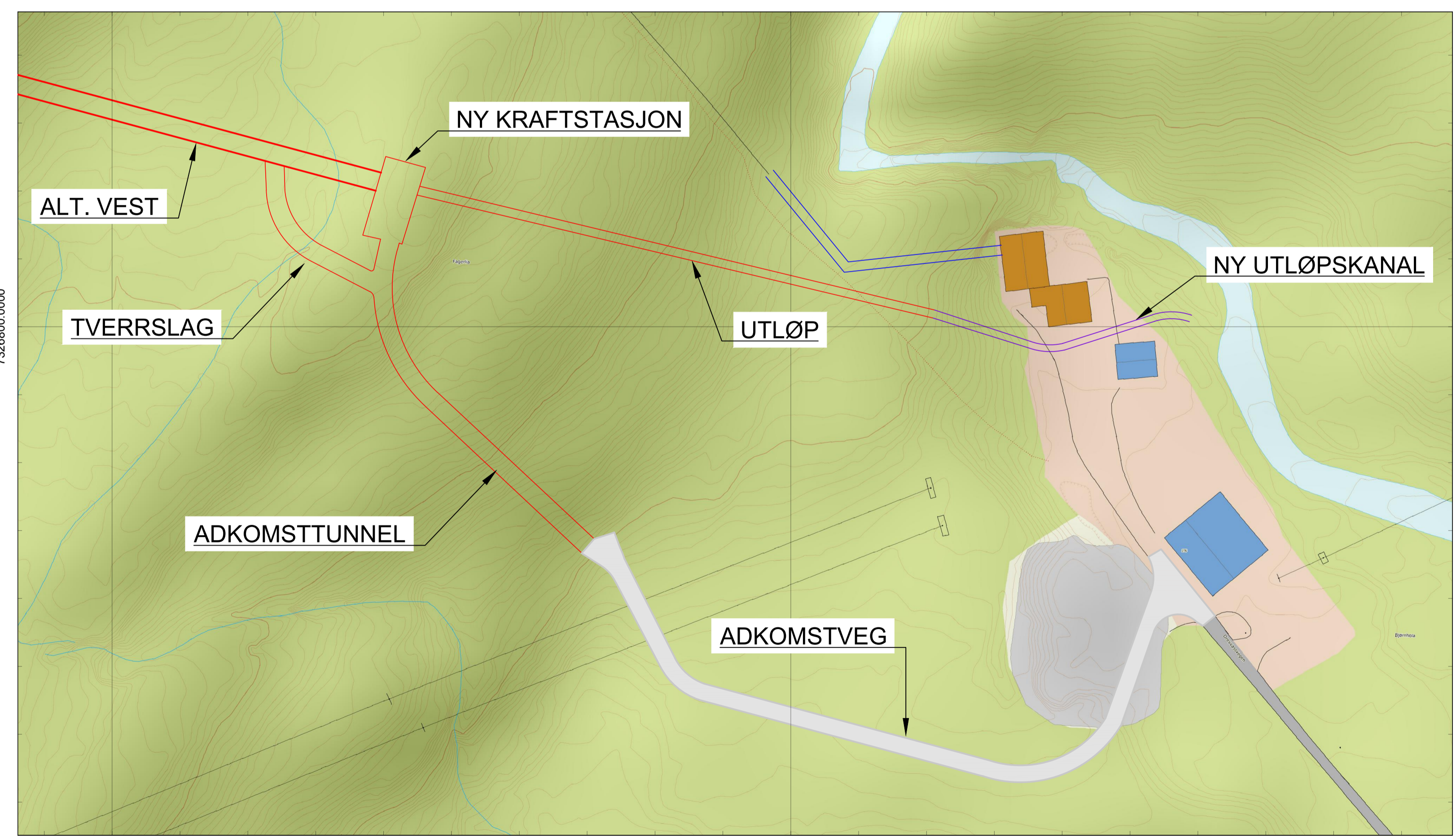
KALDÅGA KRAFTVERK - KRAFTSTASJONSOMRÅDE - STASJON I BERG - PLAN 1:1000
