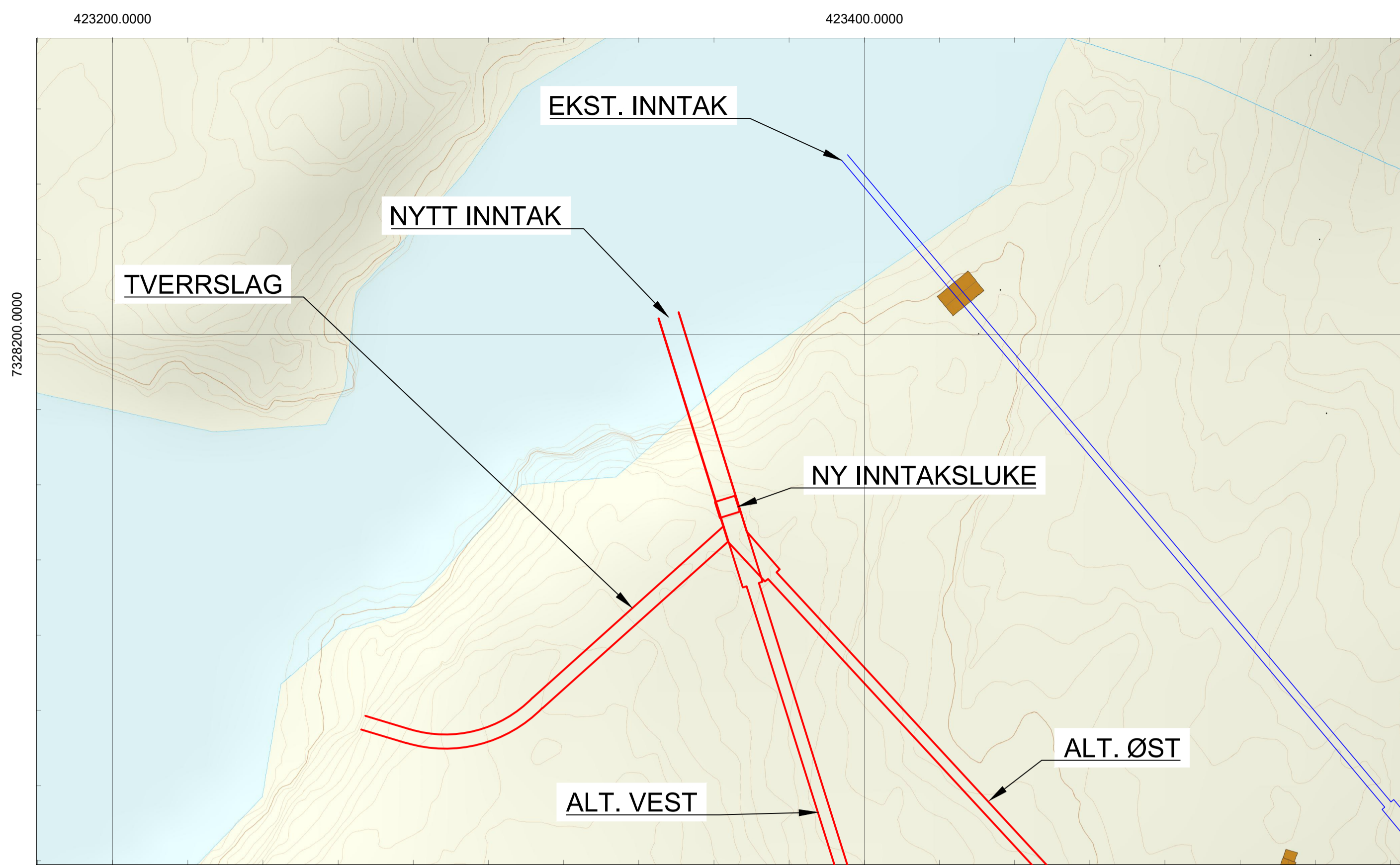
KALDÅGA KRAFTVERK - NYTT INNTAK ENVATN - PLAN 1:1000
