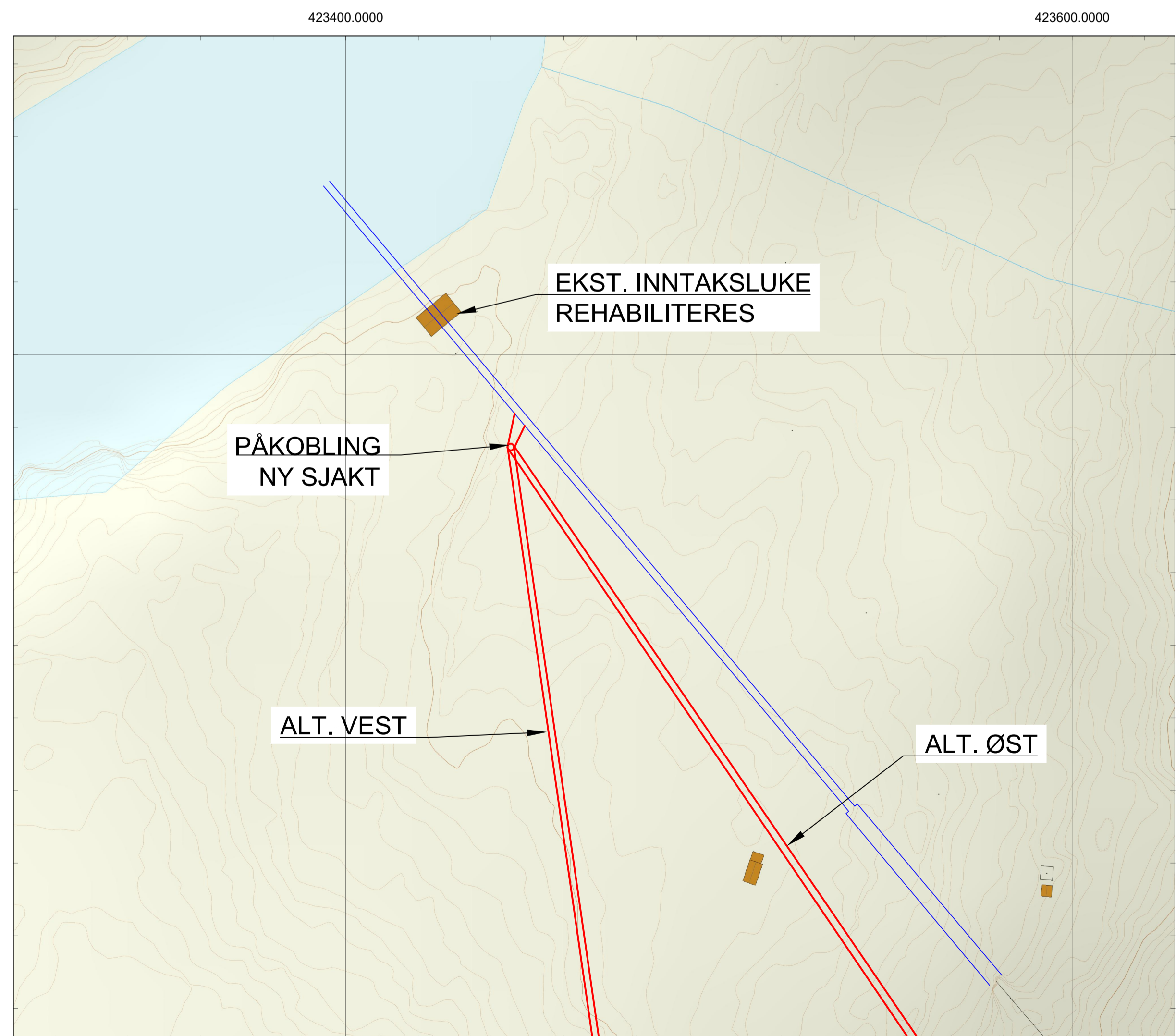
KALDÅGA KRAFTVERK - REHABILITERING INNTAK ENVATN - PLAN 1:1000
