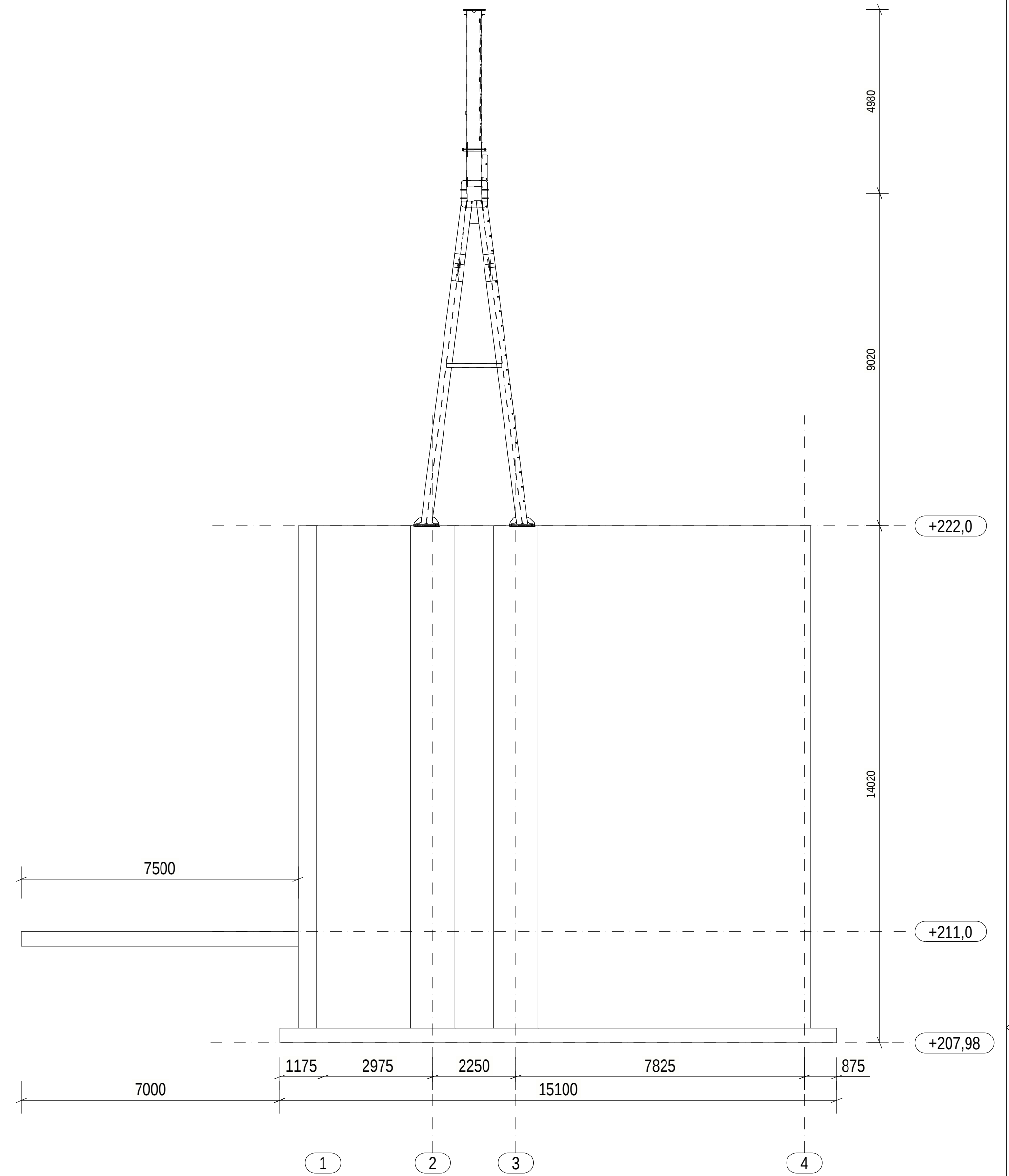
B - B 1:100
