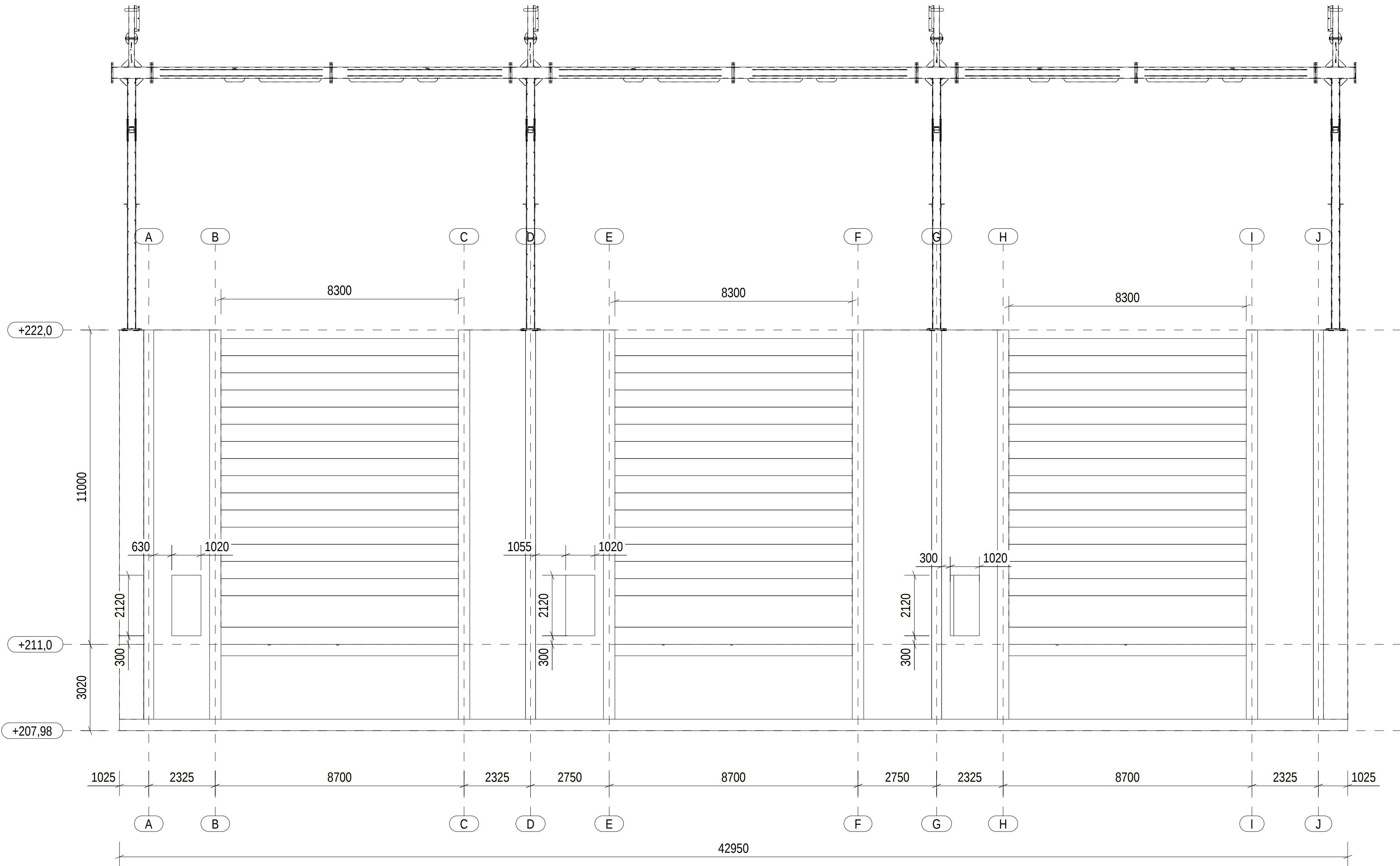
A - A 1:100
