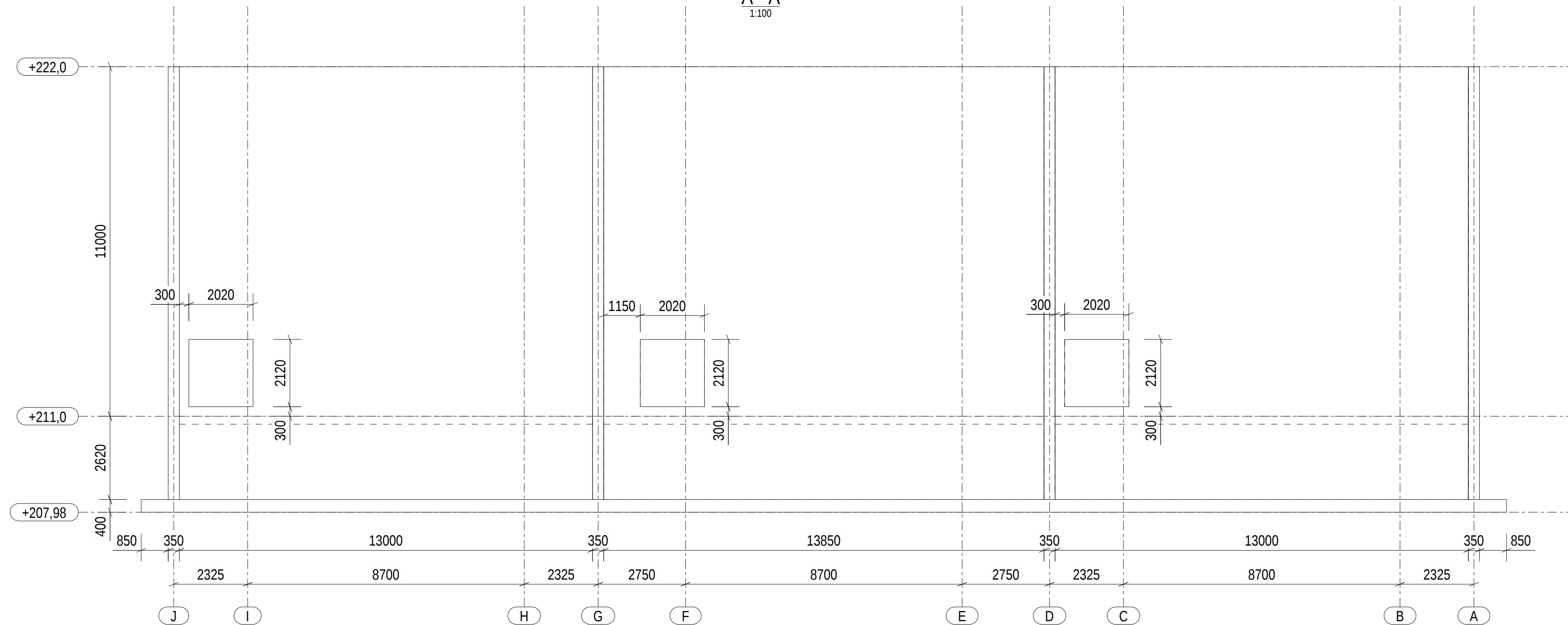
C - C 1:100
