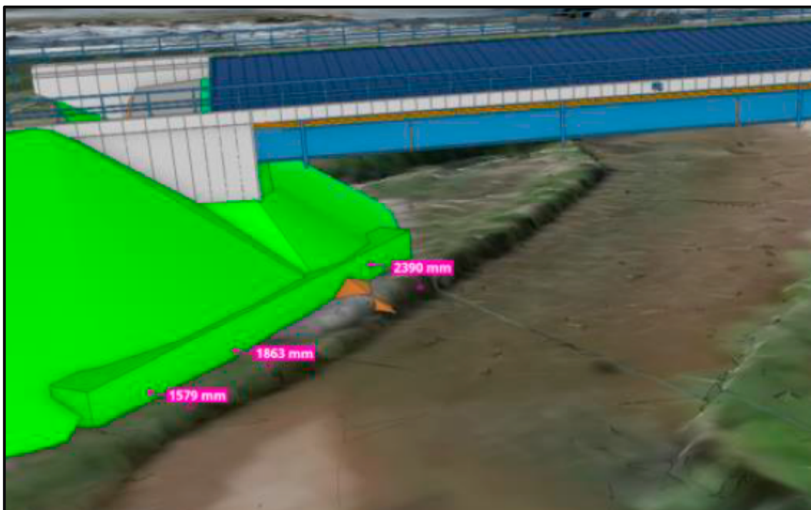
Figur 2 Illustrasjon av planlagt løsning for landkar mot Lødingen (Akse 1).
