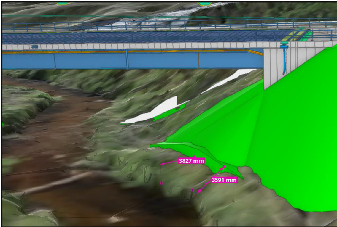
Figur 3: Illustrasjon av planlagt løsning for landkar mot Sortland (Akse 4).
