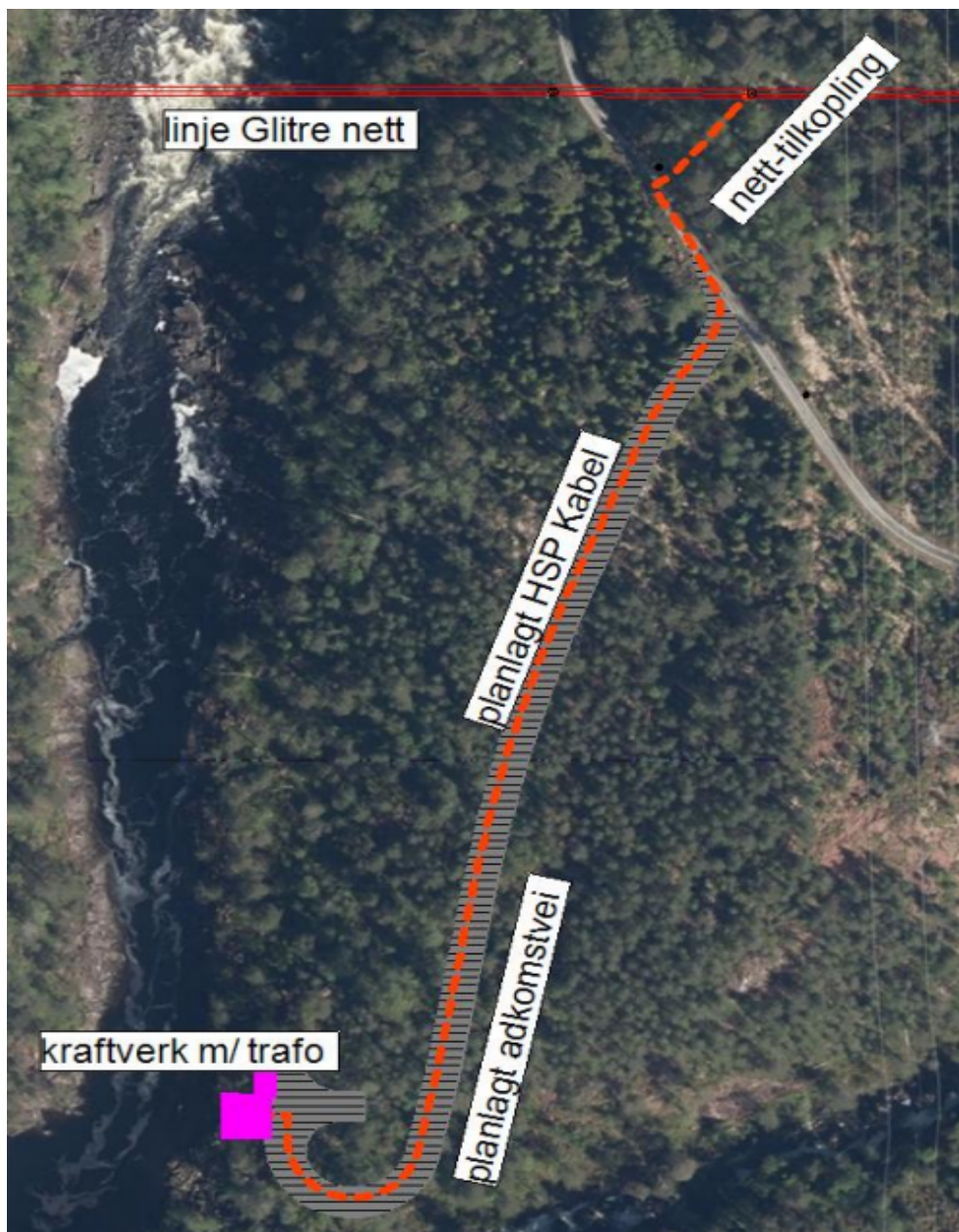
Figur 1: Gjosa kraftverk tilknyttes overliggende nett via en om lag 275 meter lang 22 kV jordkabel. Jordkabelens trasé er markert med rød stiplest strek. Kilde: Gjosa kraftverk sin søknad av januar 2025.
