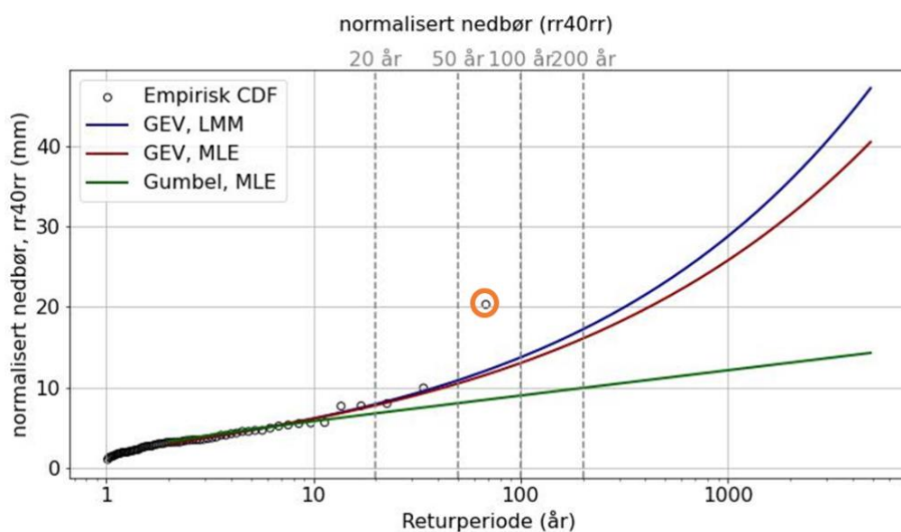
Figur 7: Ekstremverdifordeling basert på 3 ulike metoder. Observasjonen under Hans er innringet med oransje.
