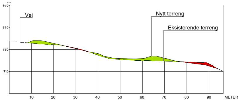
Snitt A-A'
