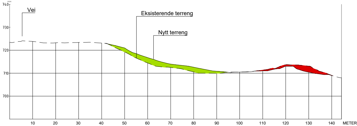
Snitt B-B'
