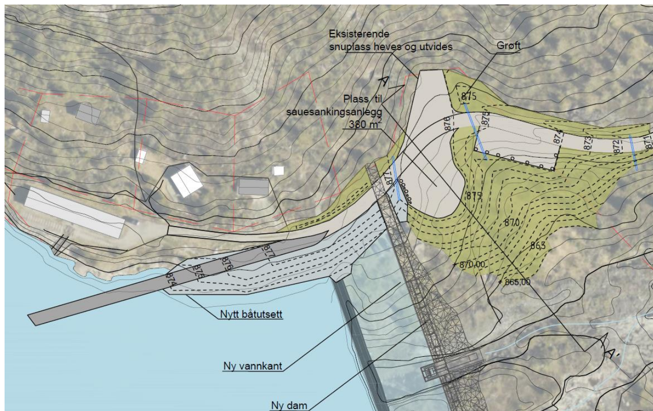
Figur 3-8 Landskapsplan for istandsetting rundt ny dam, se vedlegg 3.
