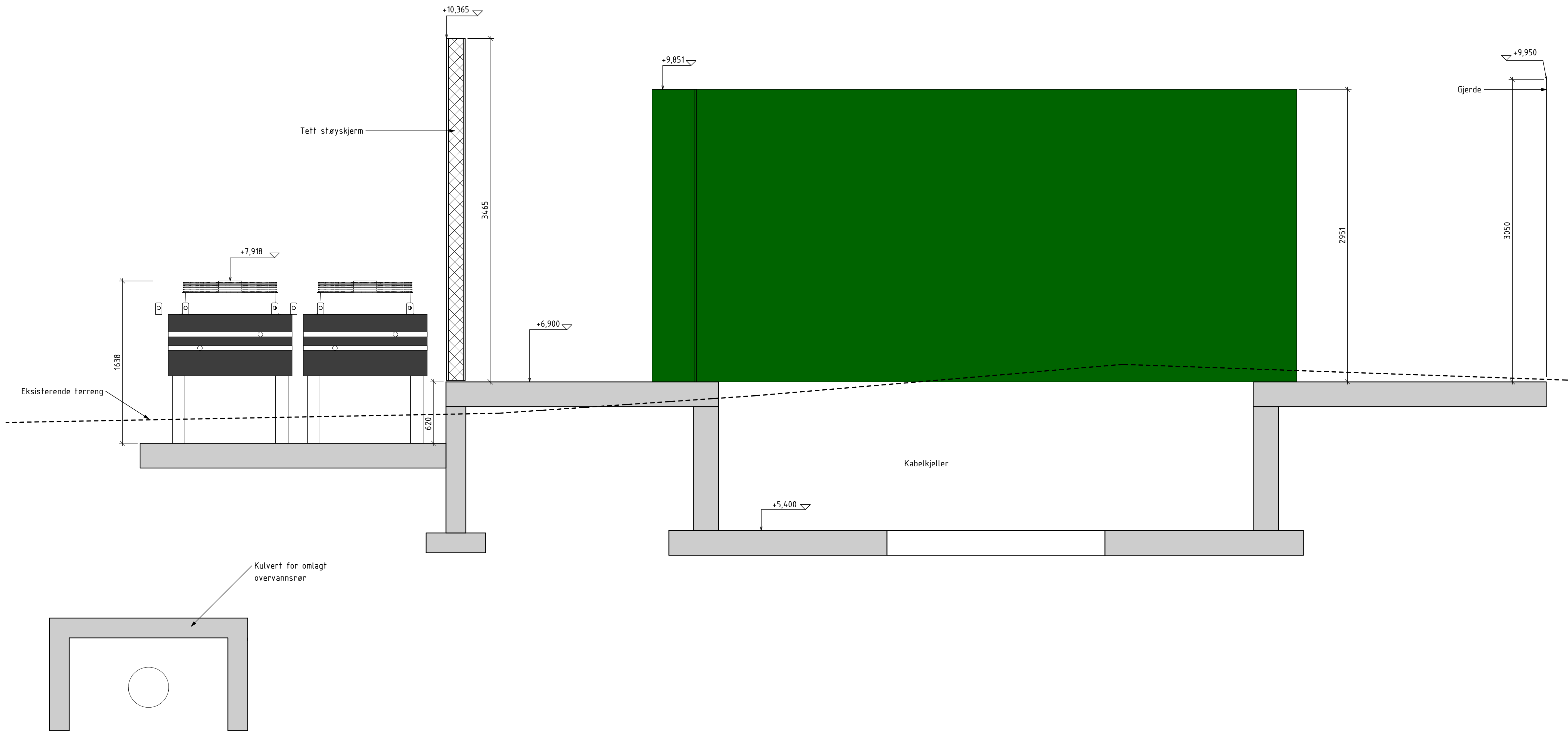
Snitt F6 Søknað 1:25
