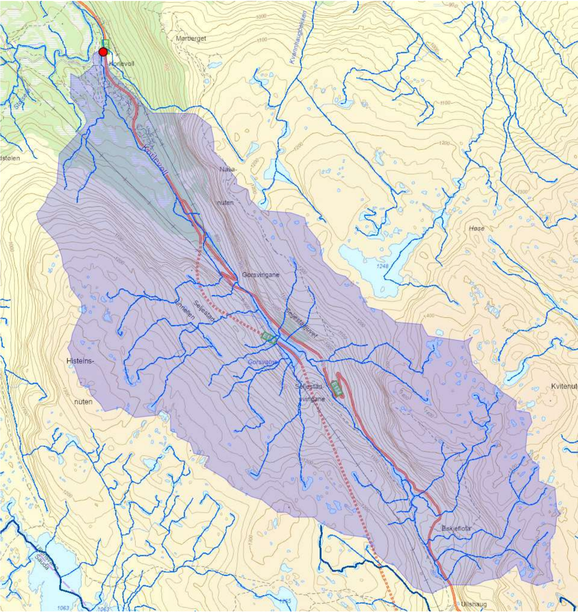
Vedlegg 2b Oversiktskart Histeinselva med nedbørfelt
