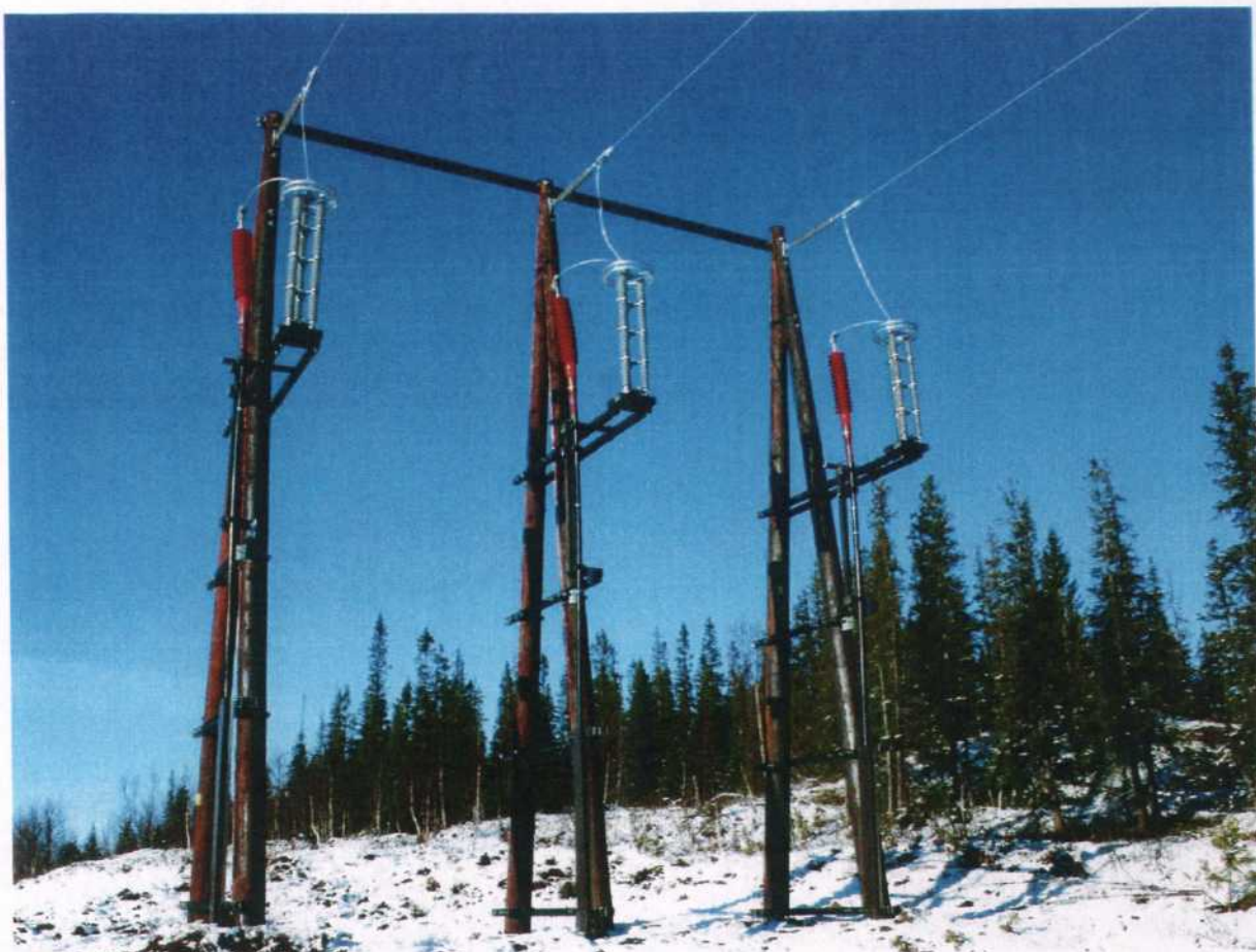
Kabelmast med avledere (Bilde gjengitt med tillatelse fra El-tjeneste AS)
