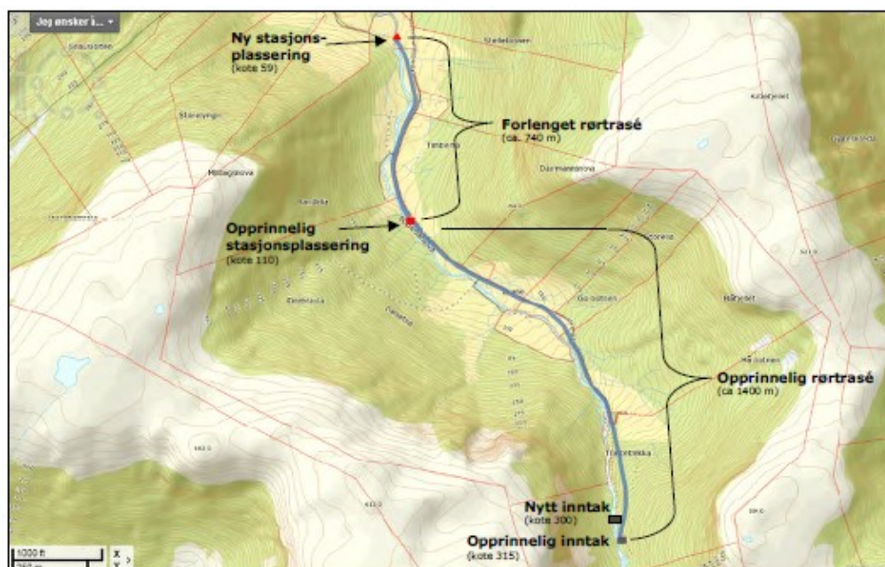
Fig. 8. Oversikt over konsesjonsgitt utbygging med inntak på kote 315, rørtrasé og stasjon på kote 110. Videre forlenget rørtrasé og ny stasjonsplassering på kote 59 og justert inntak på kote 300. Kartkilde: GisLink.
