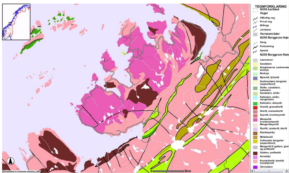
Figur 4.1 Berggrunnskart for området hvor Roan vindpark er planlagt. Kilde: Norges geologiske undersøkelse 2007 ( www.ngu.no/kart/bg250/ ).
