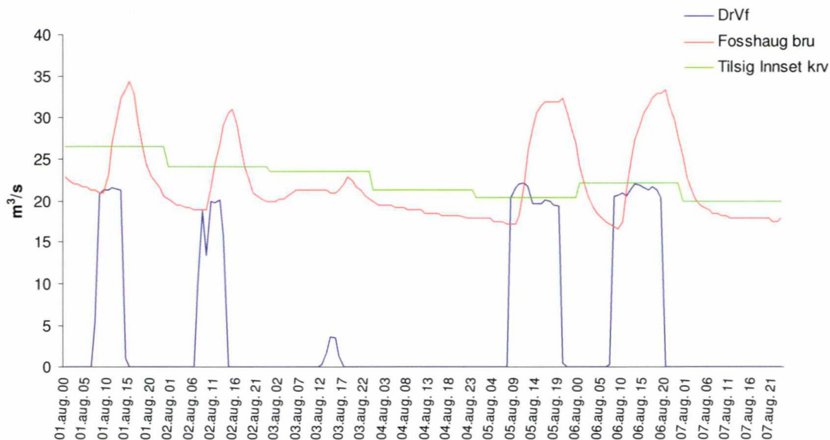
Driftsvannføring, vannføring og tilsig år 2008 1.-7. aug.
