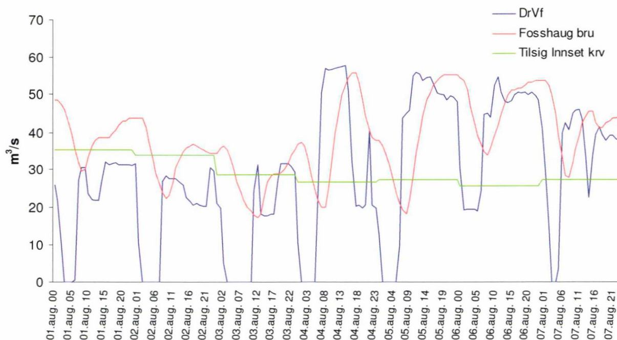
Driftsvannføring, vannføring og tilsig år 2008 1.-7. aug.
