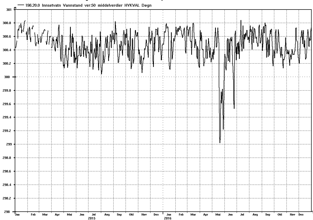
Døgnmiddelvannstand i Innsetvatn i perioden 2015-2016
