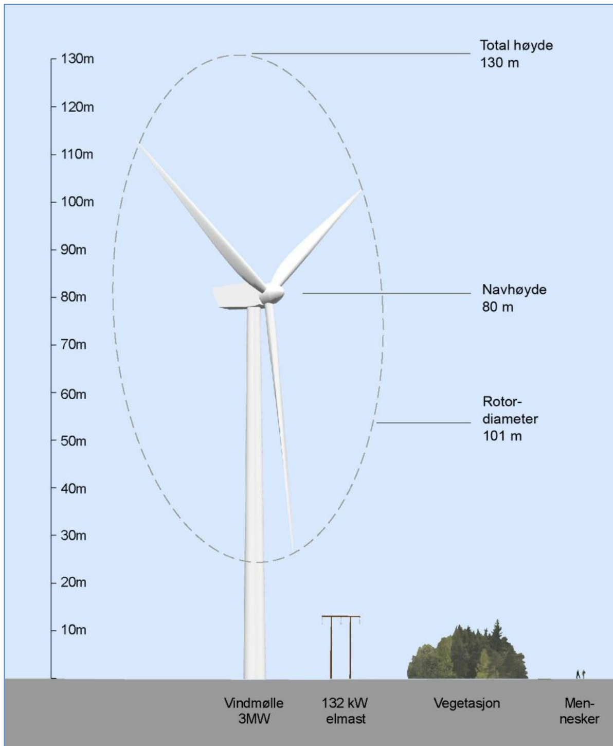
Figur 3-5. Størrelse på aktuell vindturbin sett i forhold til kraftmast, vegetasjon og mennesker. Ill.: T. Simensen, Sweco.
