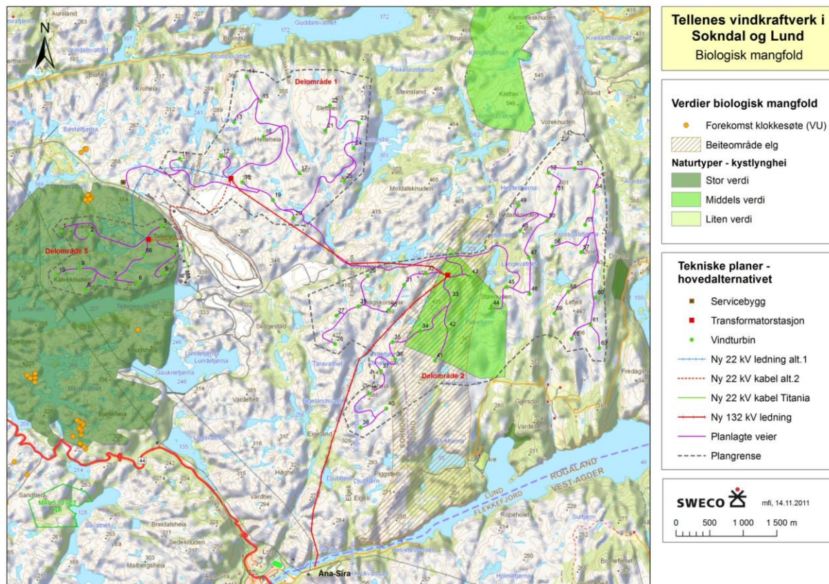
Figur 8-1. Verdisatte områder biologisk mangfold.
