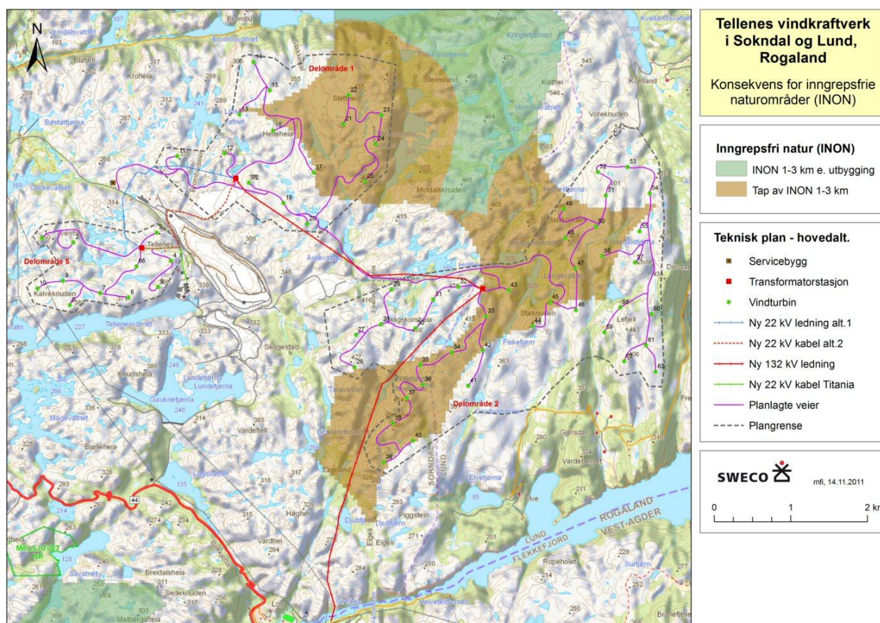
Figur 13-1. Tap av inngrepsfrie naturområder (9,37 km 2 ) er vist med brunt. Kart: Sweco.
