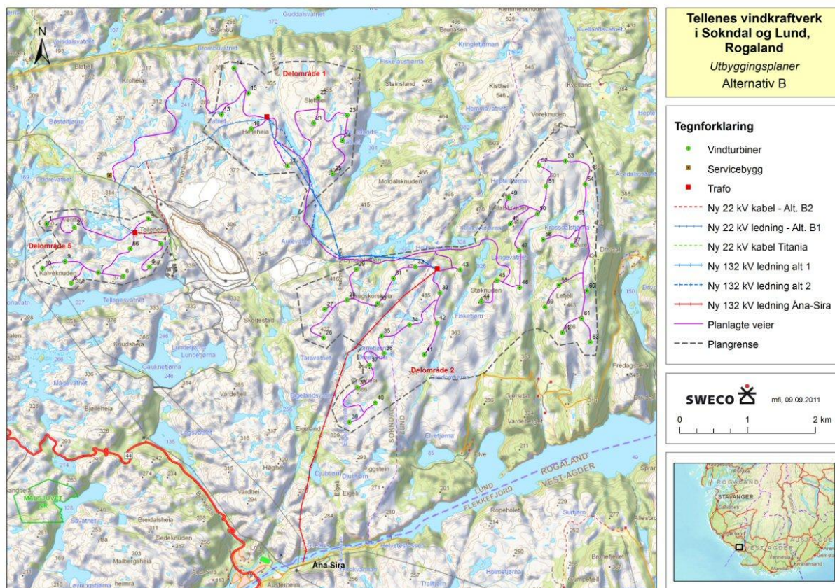
Figur 3-4. Alternativ B. Kart i større format finnes i vedlegg 2.
