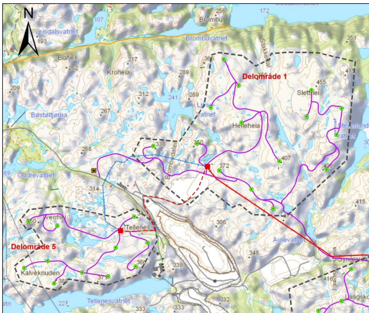
Figur 3-2. Utsnitt for delområde Tellnes 1 og 5, hovedalternativet. Det vises til tegnforklaring i Figur 3-1.
