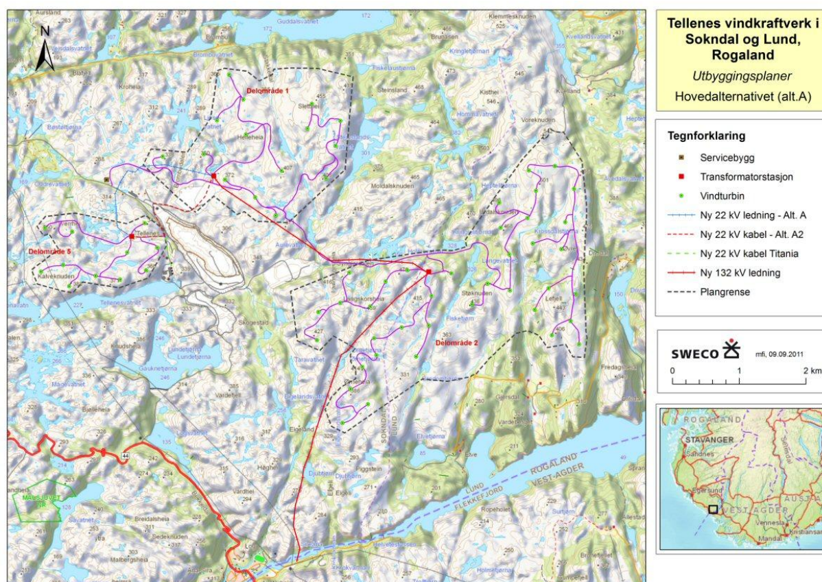
Figur 3-1. Utredet utbyggingsløsning for Tellenes vindkraftverk (hovedalternativet). Kart i større format finnes i vedlegg 2.
