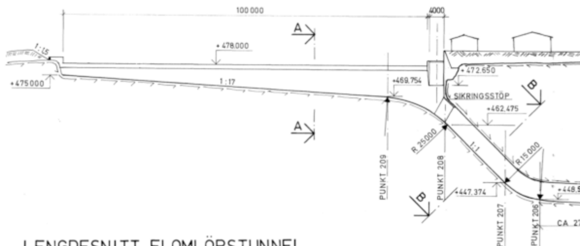
LENGDESNITT FLOMLØPSTUNNEL
