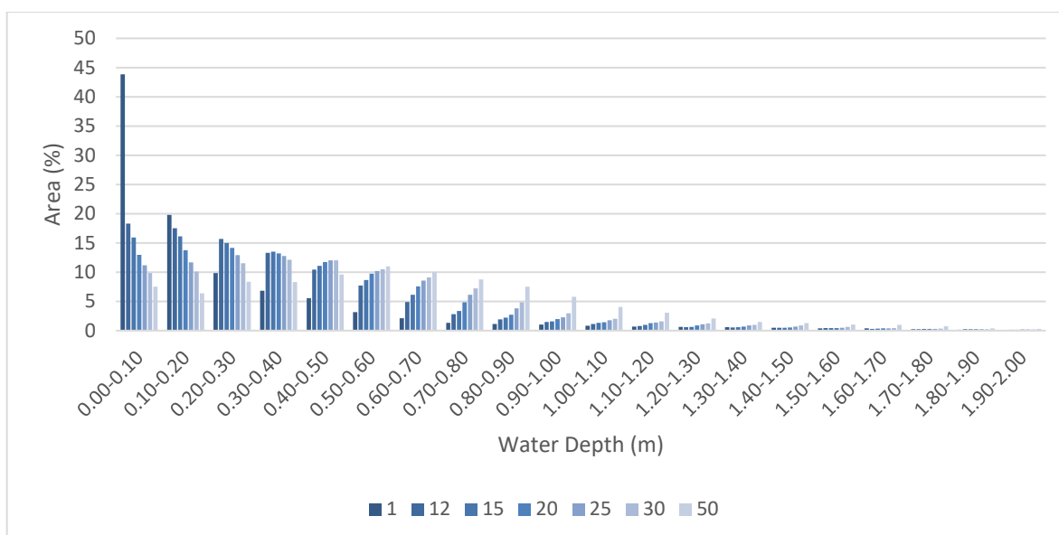
Figur 19. Vanndekt areal og vanndybde fra modellering ved Lindøy på vannføringer 1, 12, 15, 20, 30 og 50 \text{ m}^3/\text{s} .
