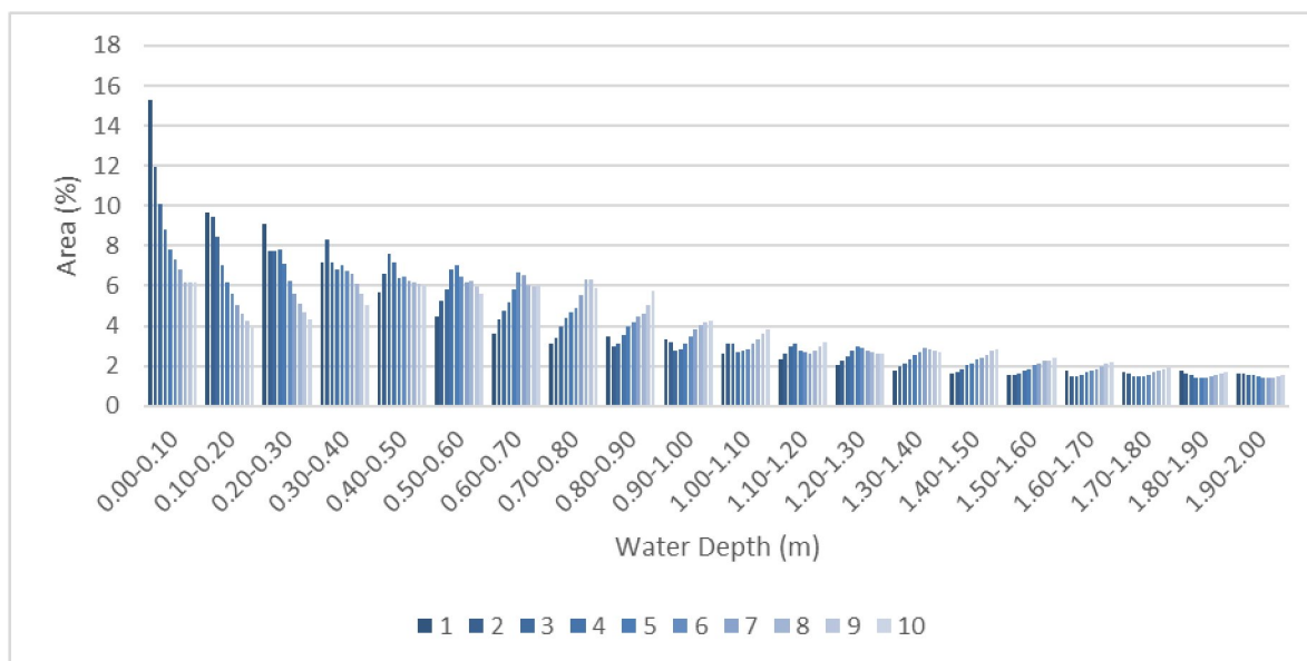
Figur 13. Arealandel med vanddybder fra modellering ved Gjesshylen på vannføringer mellom 1 – 10 \text{ m}^3/\text{s} .
