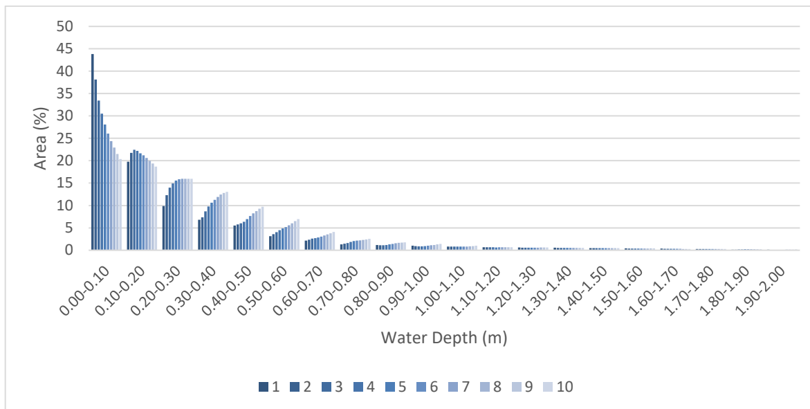
Figur 18. Vanndekt areal og vanndybde fra modellering ved Lindøy på vannføringer 1 - 10 \text{m}^3/\text{s} .
