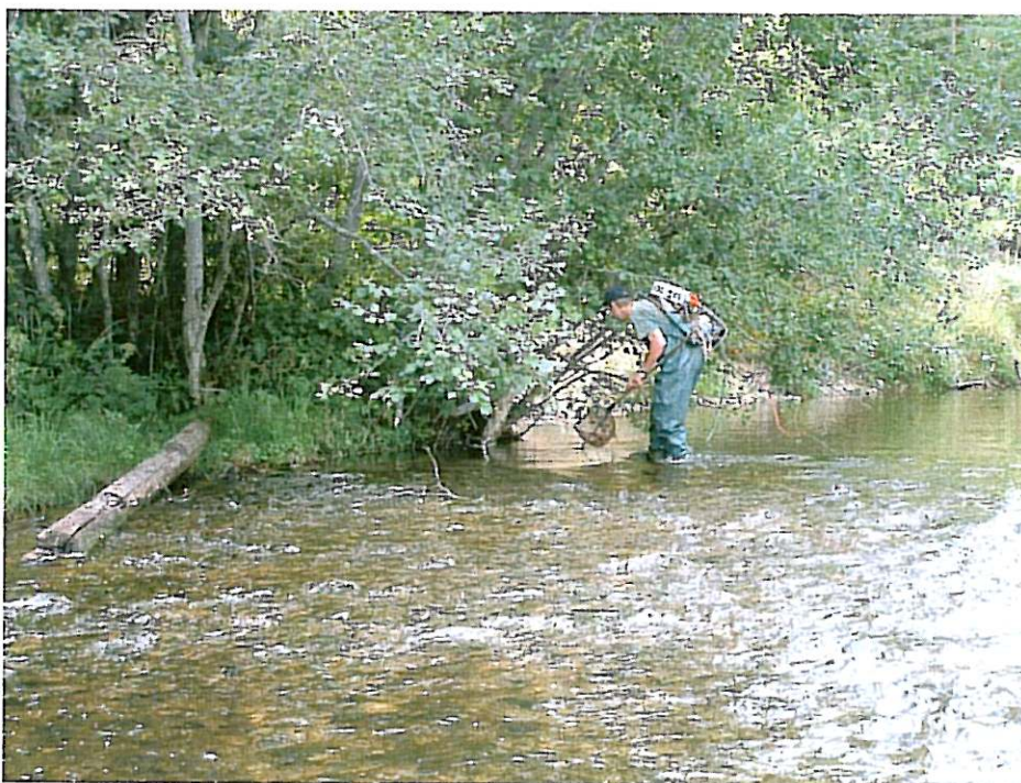
Elektrisk fiskeapparat ble benyttet i søk etter fisk i Fulldøla. Foto: Ole Roer
