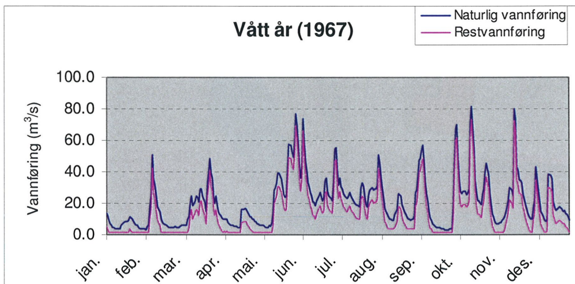
Figuren over viser restvannføringen ved Etneelva i et vått år (1967), årsavrenning på 21,21 \text{m}^3/\text{s}
