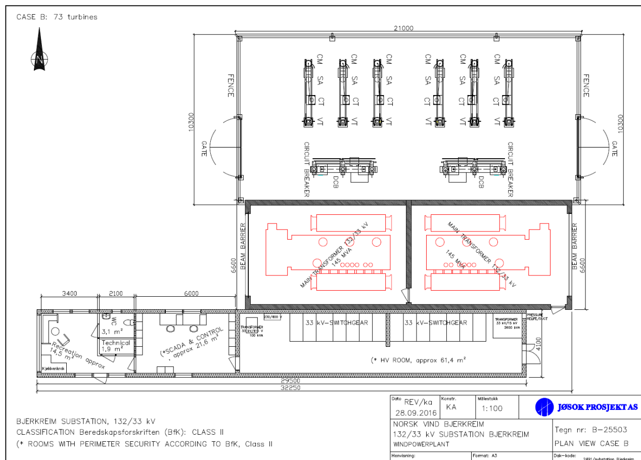
Fig. 2 Plantegning. Aktuell felles trafostasjon i Bjerkreim Vindpark (Foreløpig layout, planløsning)
