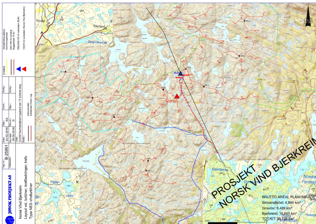
Fig. 1 Oversiktskart. 33 kV kabel layout Bjerkreim Vindpark. (Foreløpig utkast)
