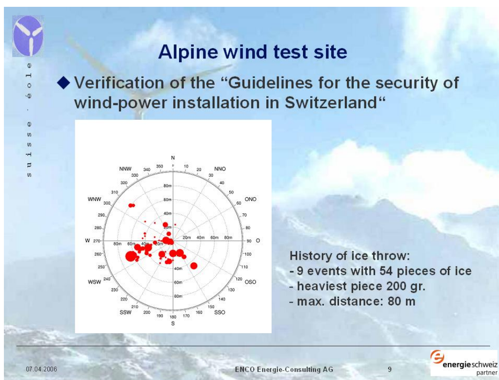
Figur 10 Resultater fra undersøkelse av iskast fra vindpark i Sveits
