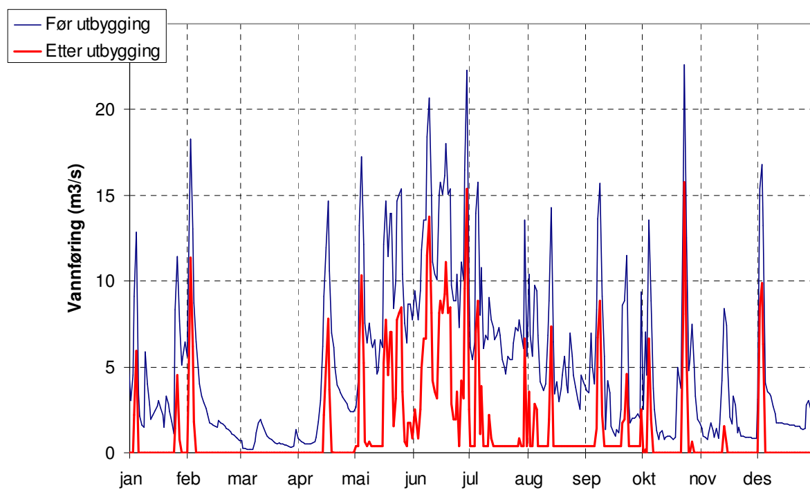
Figur 7. Plott som viser vannføringsvariasjoner i et middels (2003) år (før og etter utbygging). 17
