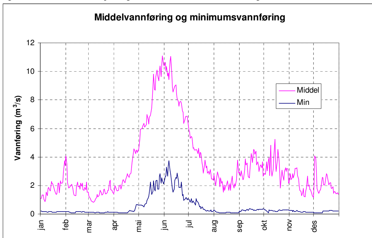
Figur 3. Plott som viser middel/median- og minimumsvannføringer (døgndata). 13
