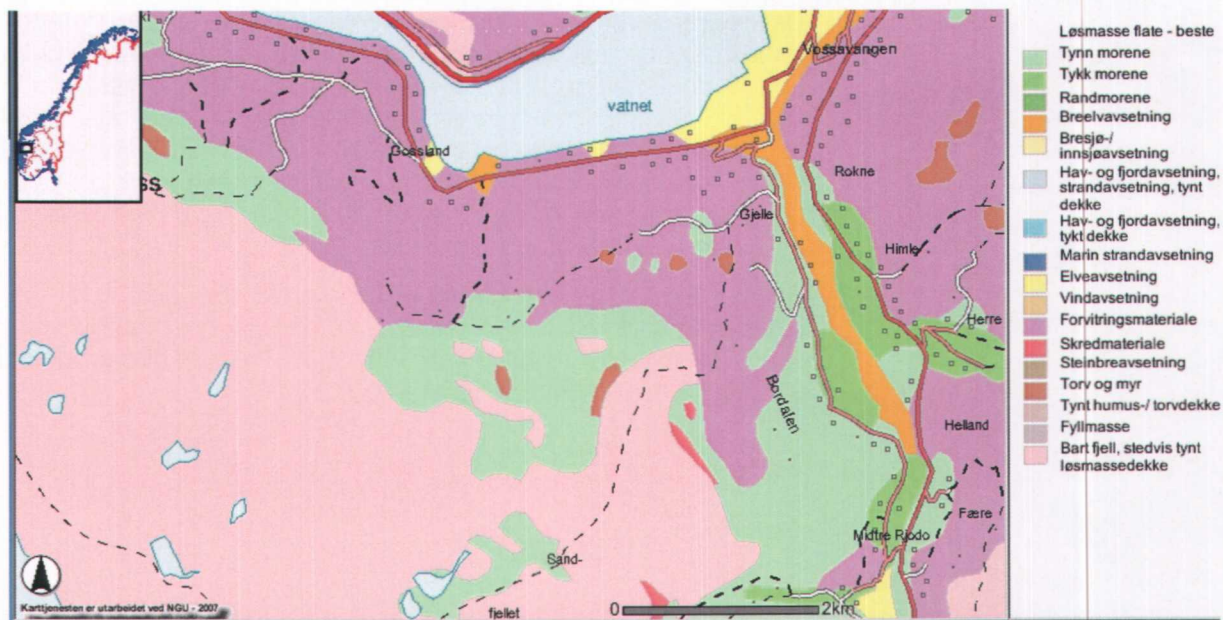
Figur 3. Det kvartærgeologiske kartet viser førekomsten av lausmassar i området kring Vangsjø og Bordalselva. Uthyggingsområdet ligg sentralt i kartutsnittet, medan Bordalselva ligg heilt til høgre. Som ein ser av kartet er det noko bre-elveavsetning ved Bordalselva, samt mykje elveavsetning ved utløpet i Vangsvatnet. (Kjelde: NGU).
