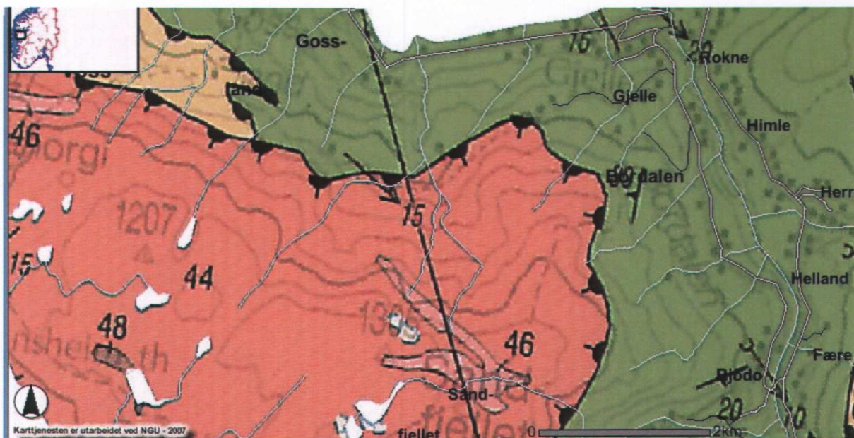
Figur 2. Dette berggrunnskartet frå området ved Vangjolo og Bordalselva viser at berggrunnen er lite variert i dette området og at det stort sett er to bergartar som dominerer. Den eine er fyllitt (den grøne), medan den andre er granitt (den raudlege).
