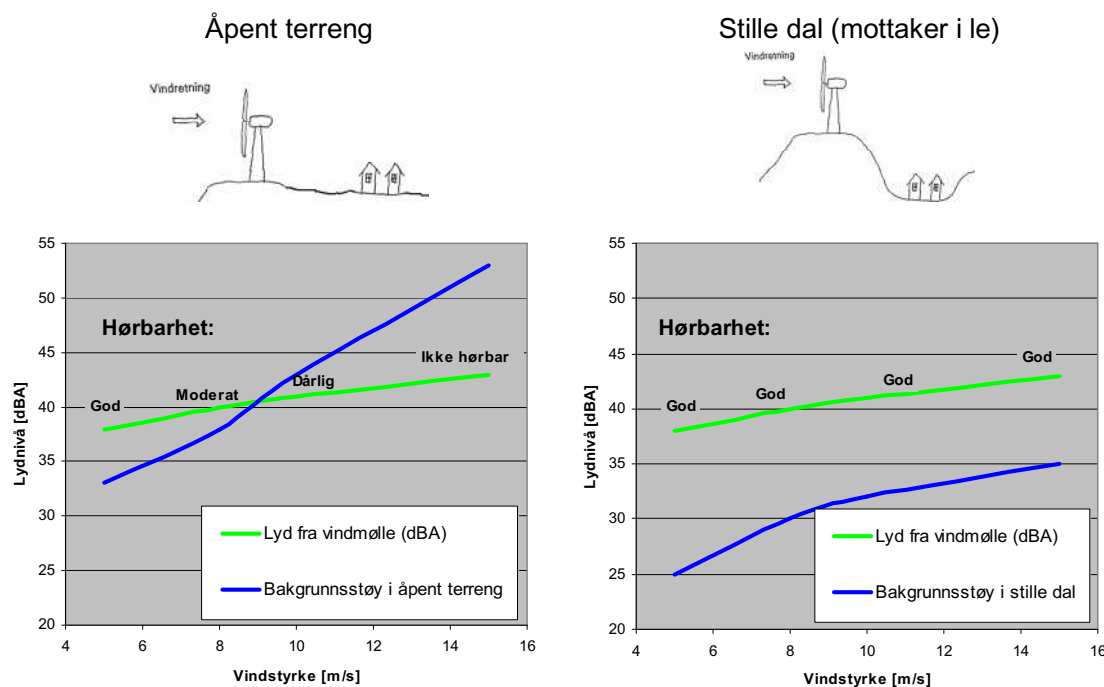
Figur 5: Eksempel på støynivåer og hørbarhet av vindturbinestøy ved ulike vindhastigheter og situasjoner. I åpent terreng maskeres lyd fra vindturbinene av bakgrunnsstøy slik at hørbarheten av turbinene blir redusert ved vind over ca 10 m/s. Hvis mottakeren befinner seg i le i en stille dal oppnås ikke denne effekten.
