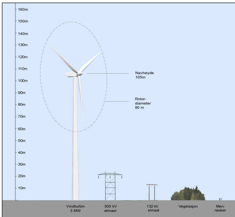
Figur 3: Skisse som viser dimensjonene på en 3 MW vindturbin sammenlignet med en 300 kV kraftledning, vegetasjon og en person. Illustrasjon: Trond Simensen, SWECO Grøner.
