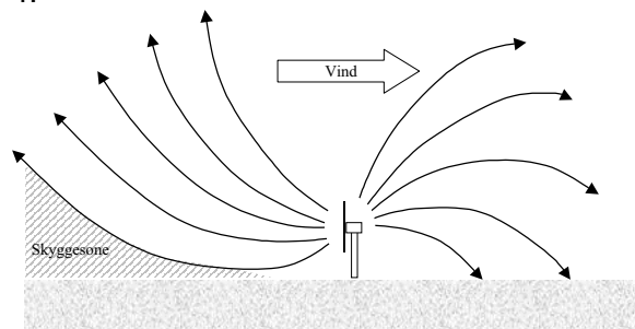
Figur 4: Innvirkning av vind på lydutbredelse.
