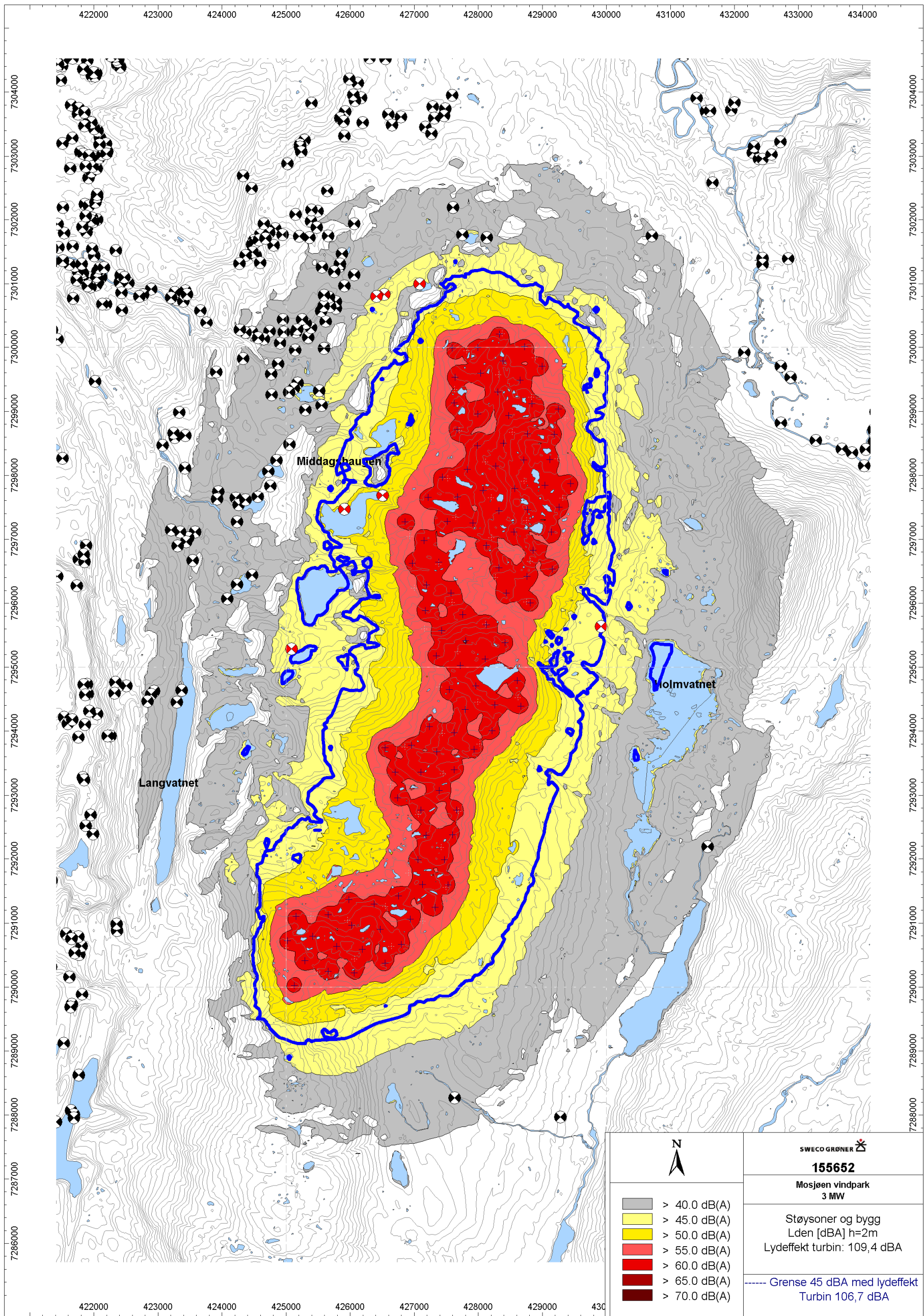
Figur 6: Driftssituasjon. 105 vindturbiner. Lydeffektnivå 109,4dBA re 1pW. Årsmidlet døgnveid lydnivå Lden korrigert for 80% driftstid. Boliger som ligger i vindskygge mer enn 30% av et normalår har grenseverdi 45 dB(A) og bør ligge utenfor gul og rød sone. Boliger/hytter med nivå over 45 dB(A) er vist med rødt. Blå linje viser hvor grensen på 45 dBA overskrides dersom det benyttes en vindturbin med lydeffekt 106,7 dBA (se Tabell 3).
