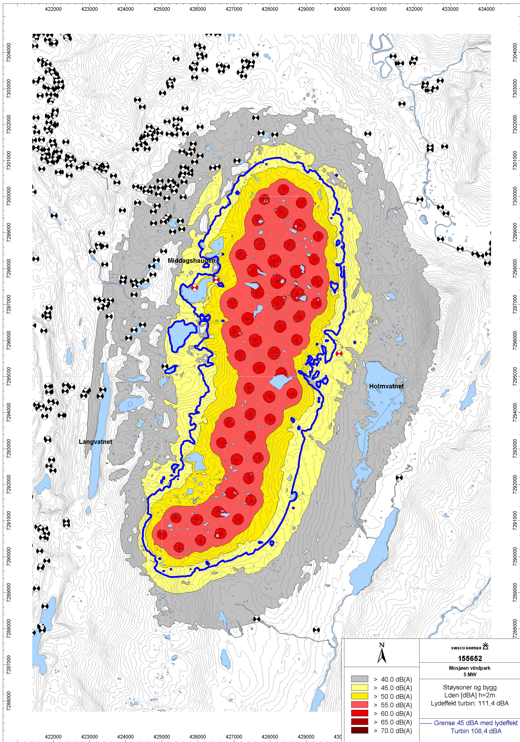
Figur 7: Driftssituasjon. 52 vindturbiner. Lydeffektnivå 111,4dBA re 1pW. Årsmidlet døgnsveid lydnivå Lden korrigert for 80% driftstid. Boliger som ligger i vindskygge mer enn 30% av et normalår har grenseverdi 45 dB(A) og bør ligge utenfor gul og rød sone. Boliger/hytter med nivå over 45 dB(A) er vist med rødt. Blå linje viser hvor grensen på 45 dBA overskrides dersom det benyttes en vindturbin med lydeffekt 108,4 dBA.
