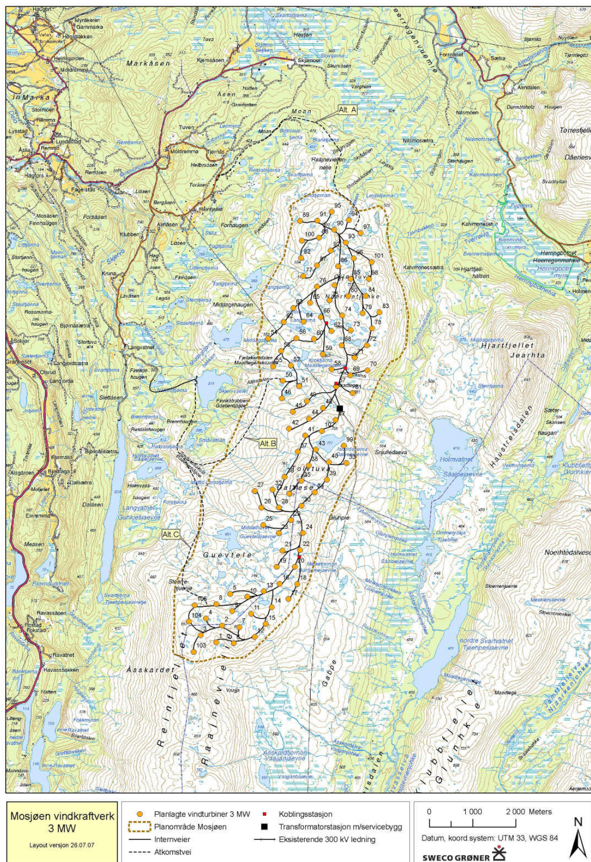
Figur 1: Mosjøen vindkraftverk. Kart over utredet 3 MW alternativ med turbiner, internveier, adkomstvei og nettløsning.
