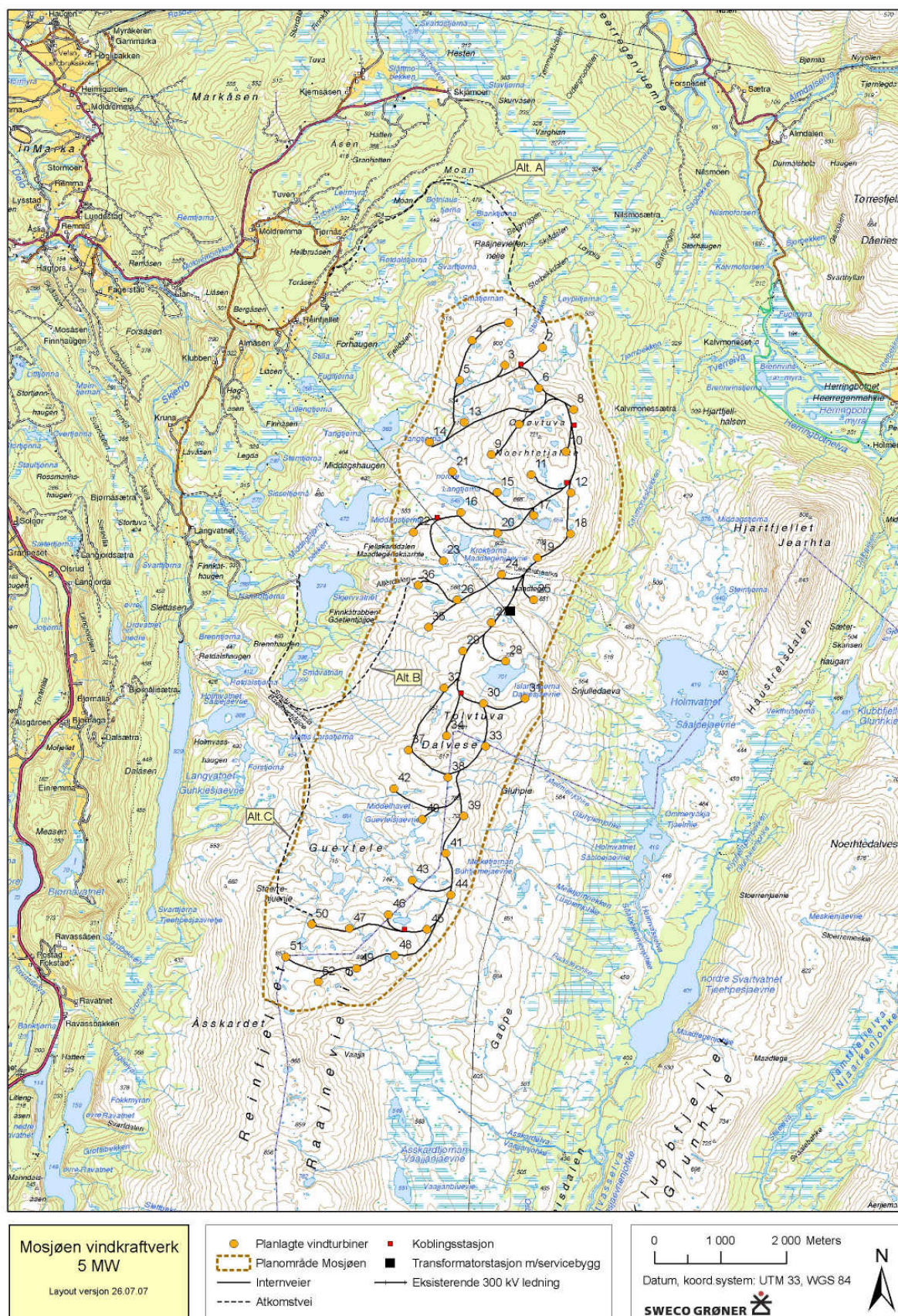
Figur 2: Mosjøen vindkraftverk. Kart over utredet 5 MW alternativ med turbiner, internveier, adkomstvei og nettløsning.
