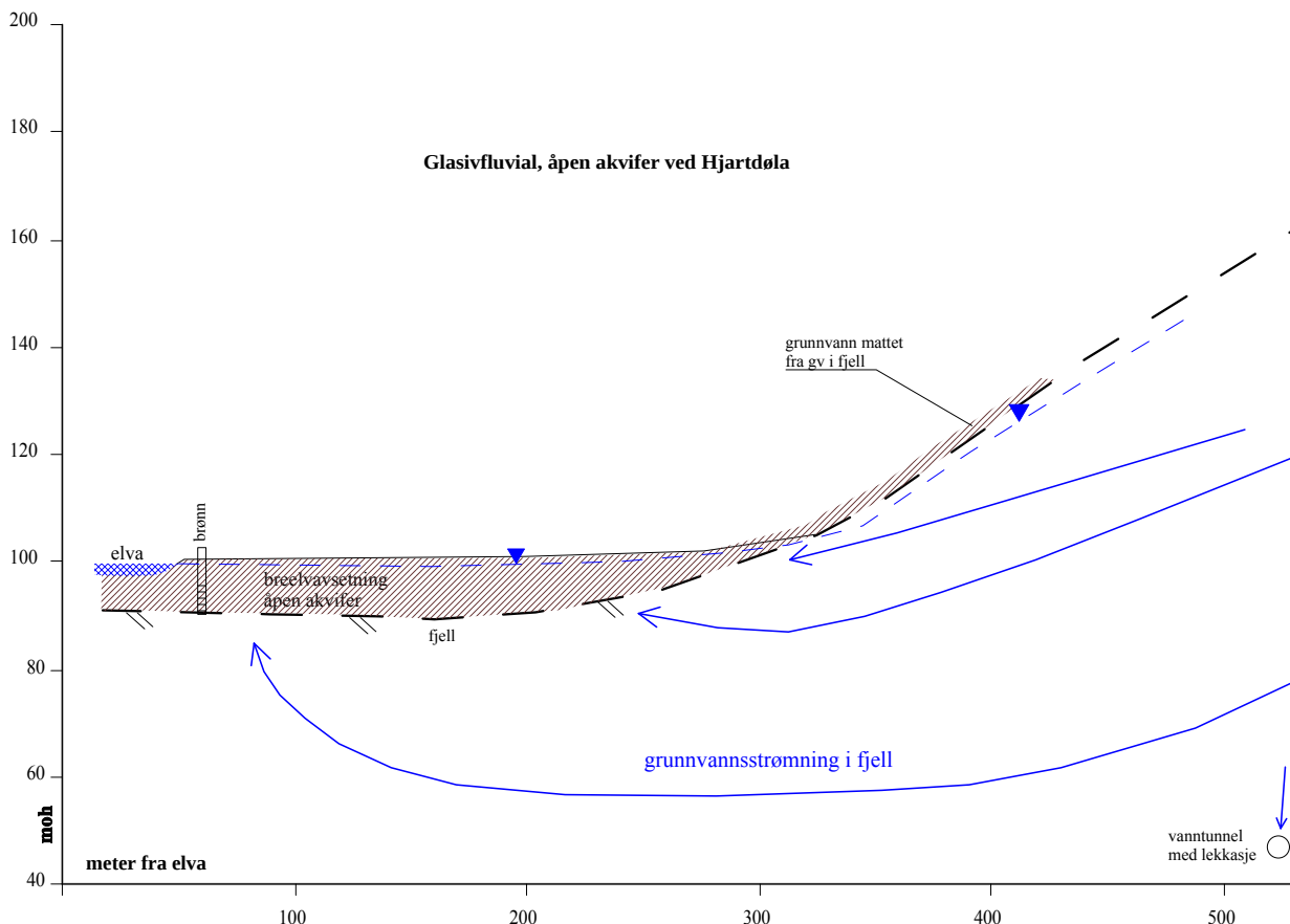
Figur 5 Åpen akvifer ved Hjartdøla og nedre seksjon av Skogsåa. Vanntunnelen er illustrativ og vertikalplassering stemmer ikke med planer.
