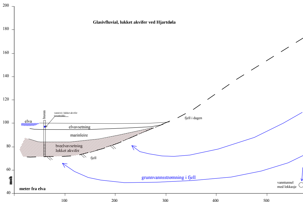
Figur 4 Lukket grunnvannsmagasin (akvifer) ved Hjartdøla, (av den typen som Sauland vannverk tapper). Vanntunnelen er illustrativ og vertikalplassering stemmer ikke med planer.
