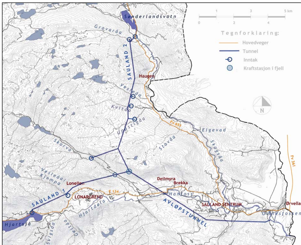
Figur 2 Prosjektområdet Sauland Kraftverk.
