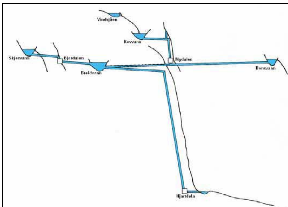
Figur 2.2. Eksisterende magasin og kraftverk i Hjordøla- og Tuddalsvassdraget
