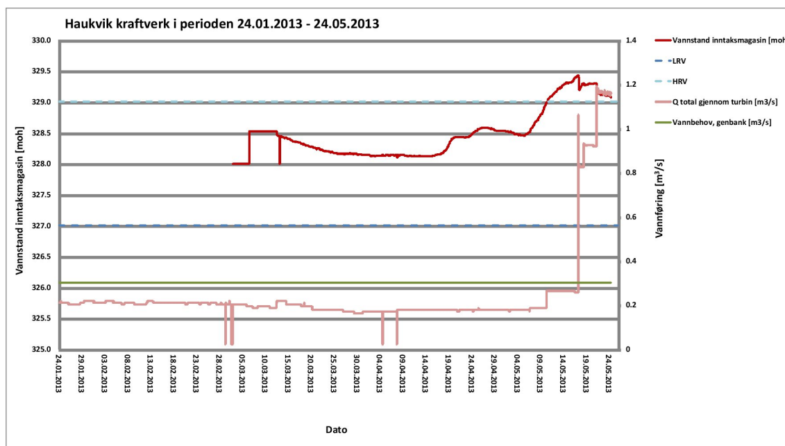
Figur 1 og 2 Sammenheng mellom vannstand i inntaksmagasin, vannforbruk i kraftstasjon og optimalt vannbehov i genbanken
